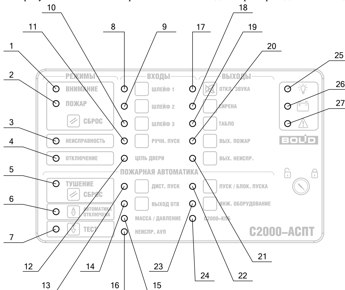
Рисунок 1. Расположение световых индикаторов
