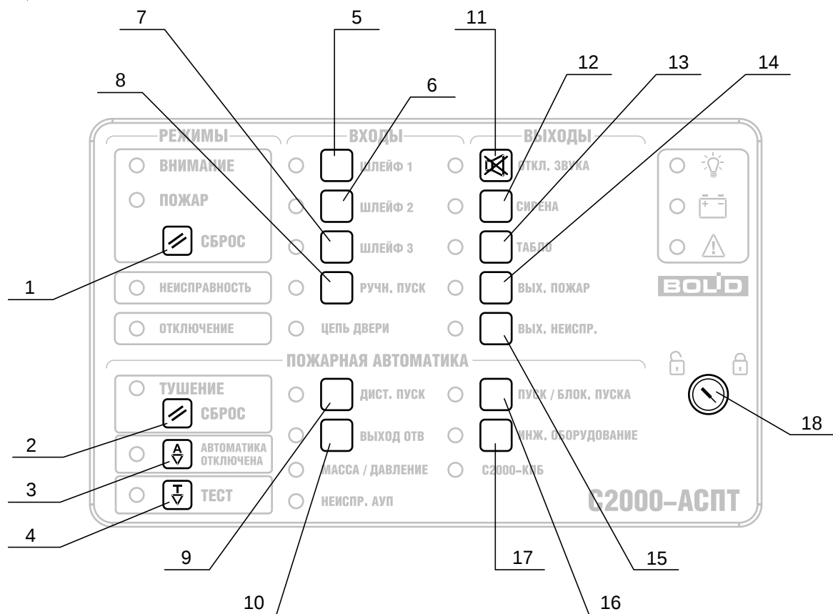
Рисунок 2. Расположение кнопок
