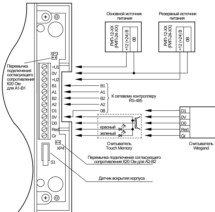
Рисунок 3. Схема внешних соединений блока «С2000-БИ 2RS485», «С2000-БИ исп.02 2RS485»
