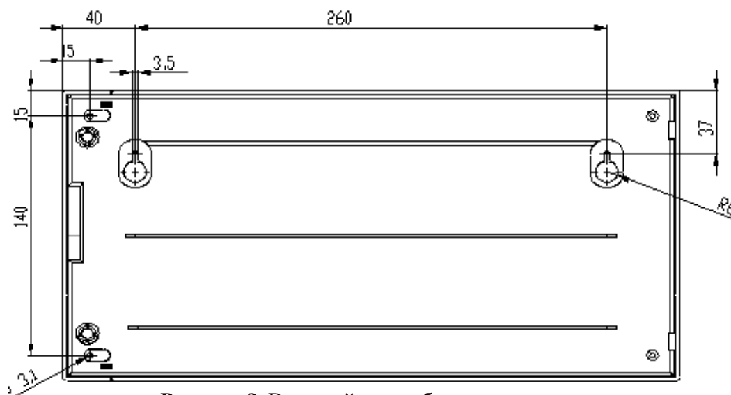
Рисунок 2. Внешний вид, габаритные и установочные размеры блока
