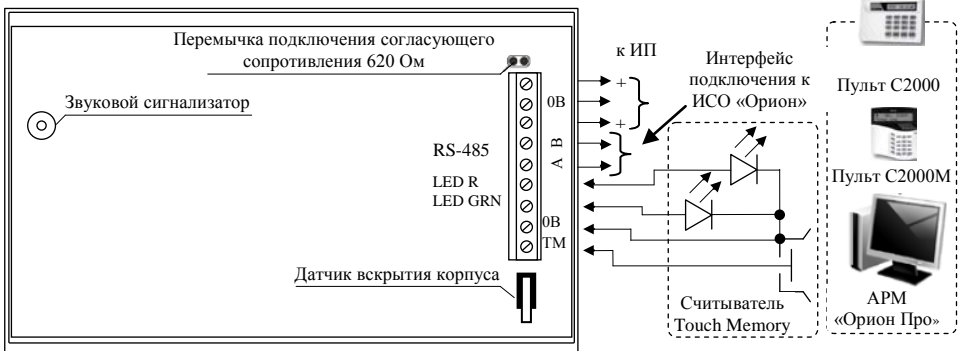
Рисунок 3. Схема внешних соединений блока «С2000-БКИ» АЦДР.426469.030 ЭТ Изм.16 АЦДР.6040-17 от 06.10.2017
