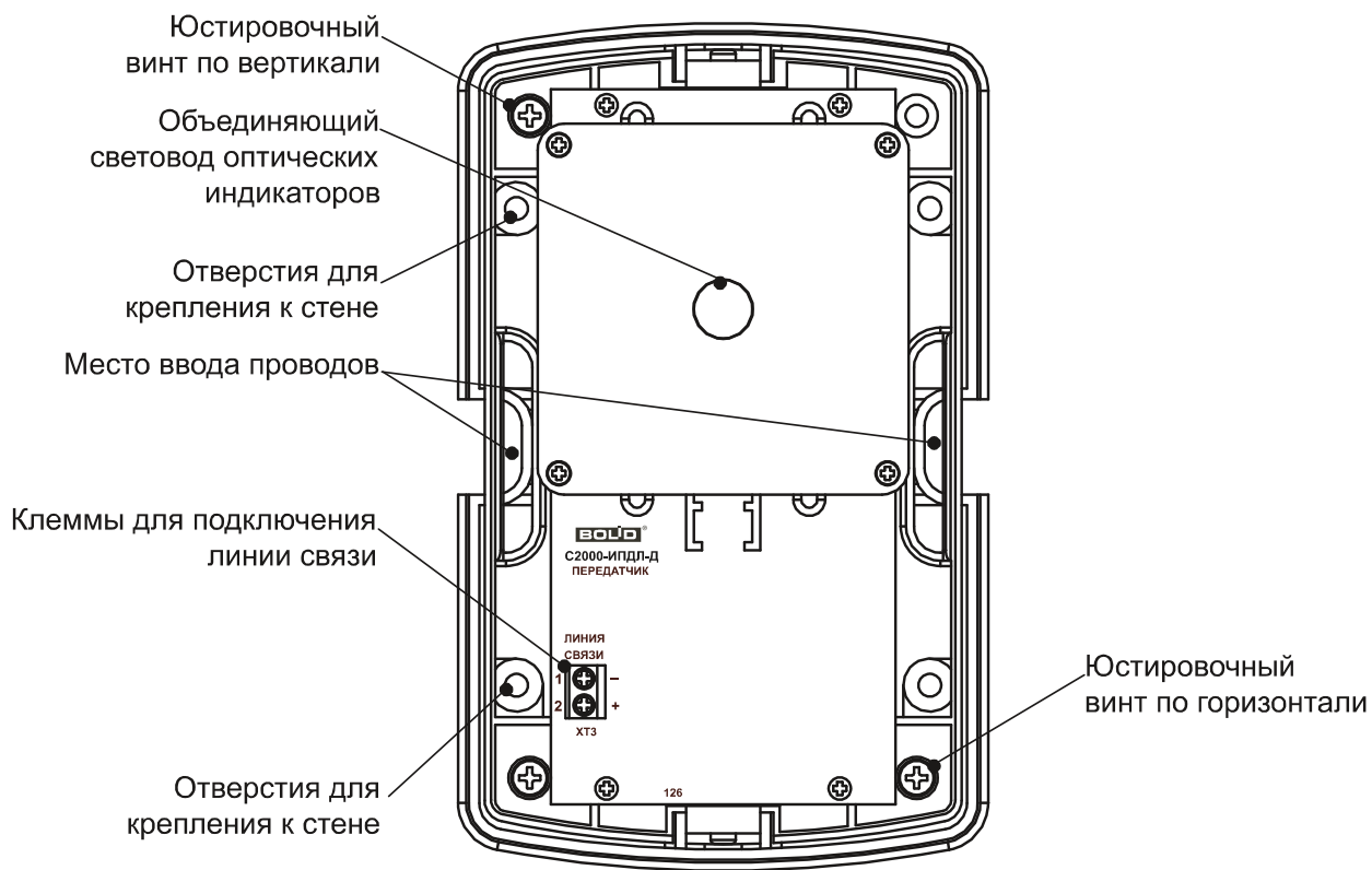
Рисунок 2.2.3.3.2 (Передатчик)
