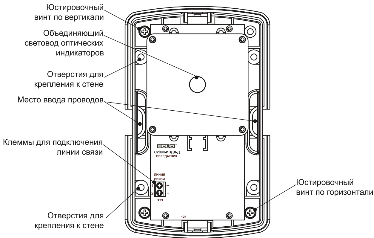
Рисунок 2.2.3.3.2 (Передачик)
