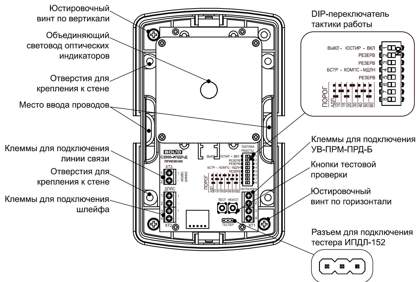
Рисунок 2.2.3.3.1 (Приемник)
