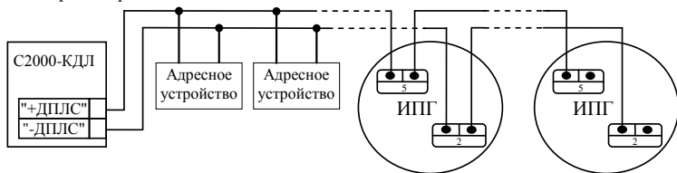
Рисунок 1. Схема соединений
