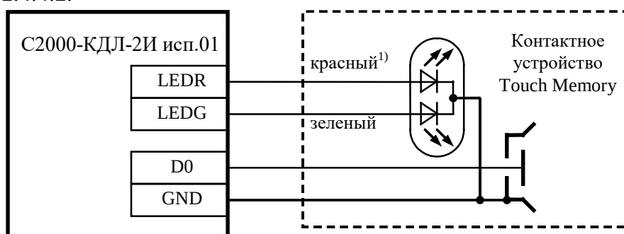
Рисунок 2.2.4.4.1 Схема подключения контактного устройства Touch Memory
