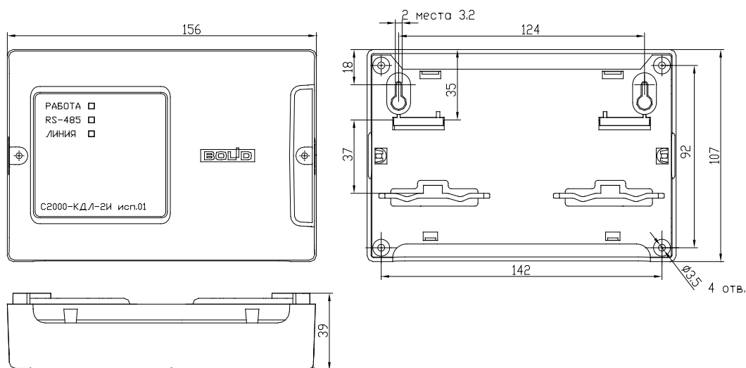
Рисунок 2.2.2.1. Габаритные и установочные размеры контроллера
