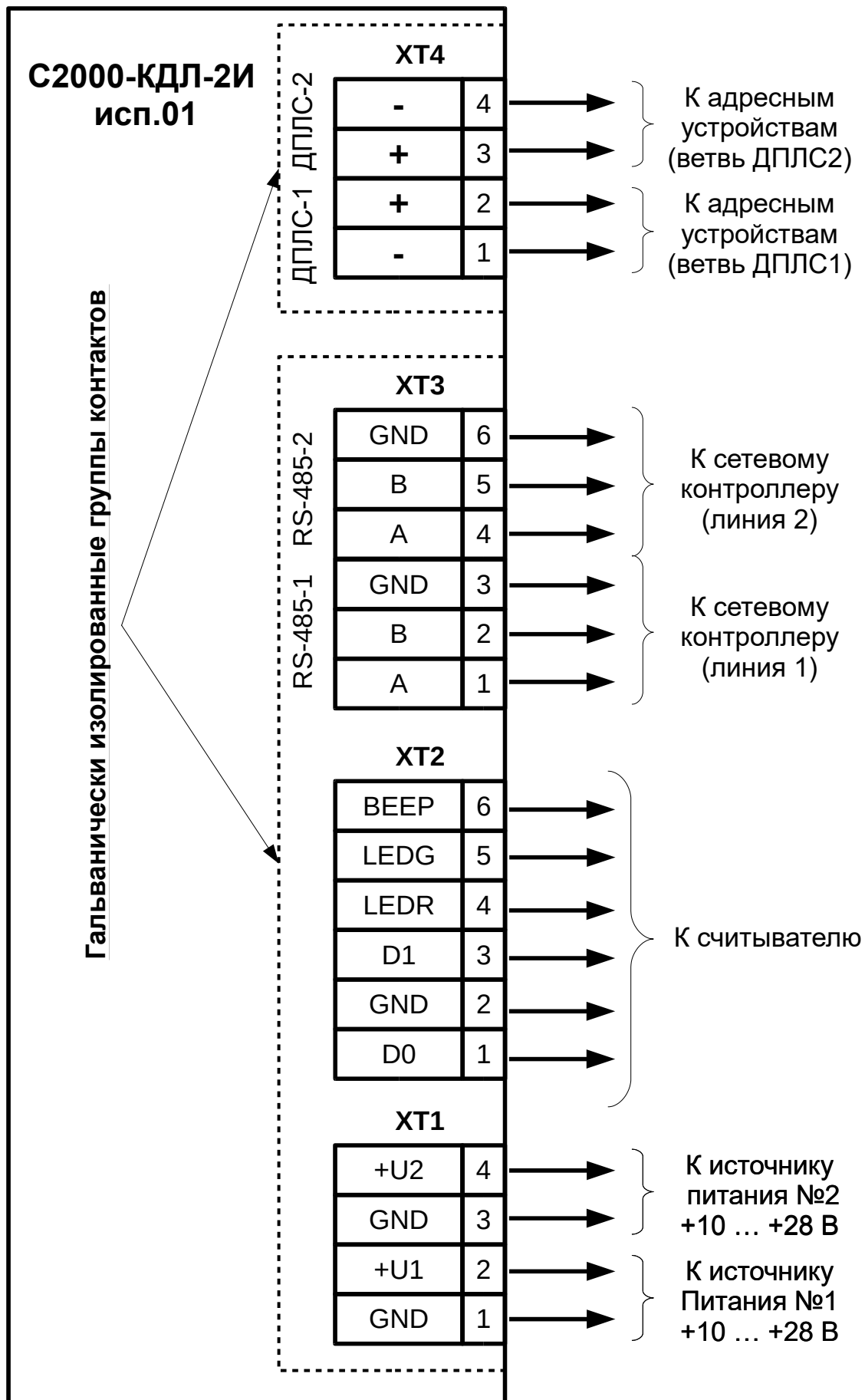
Рисунок 2.2.4.1. Схема электрическая подключения контроллера
