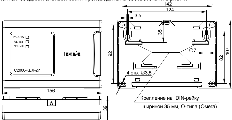
Рисунок 1. Габаритные и установочные размеры контроллера
