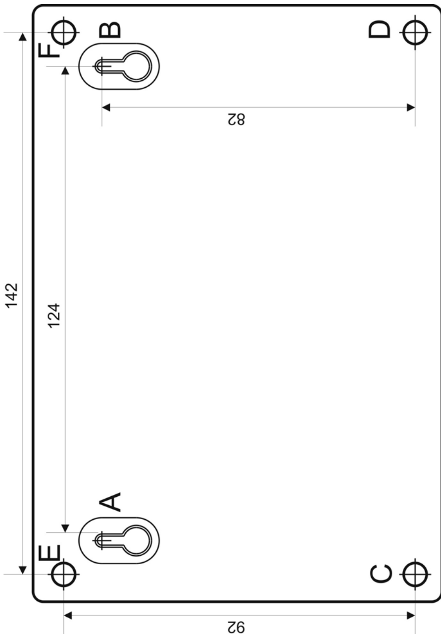
Рисунок 10. Шаблон для монтажа
