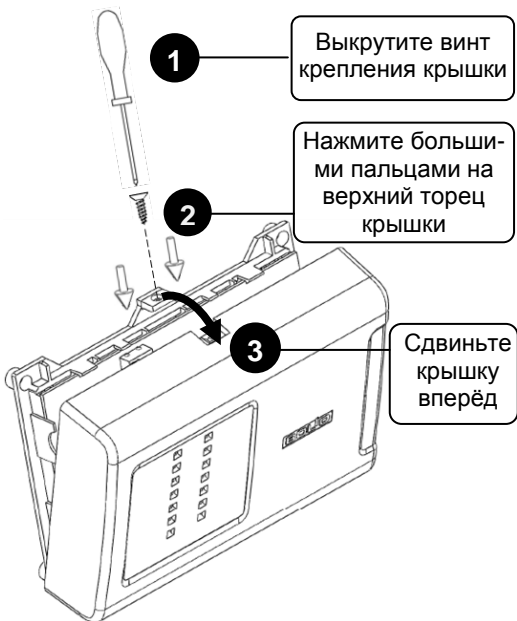
Рисунок 2. Снятие крышки контроллера
