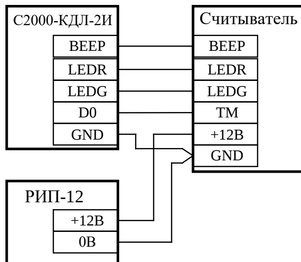
Рисунок 2.2.4.4.2. Схема подключения считывателей с интерфейсом Touch Memory
