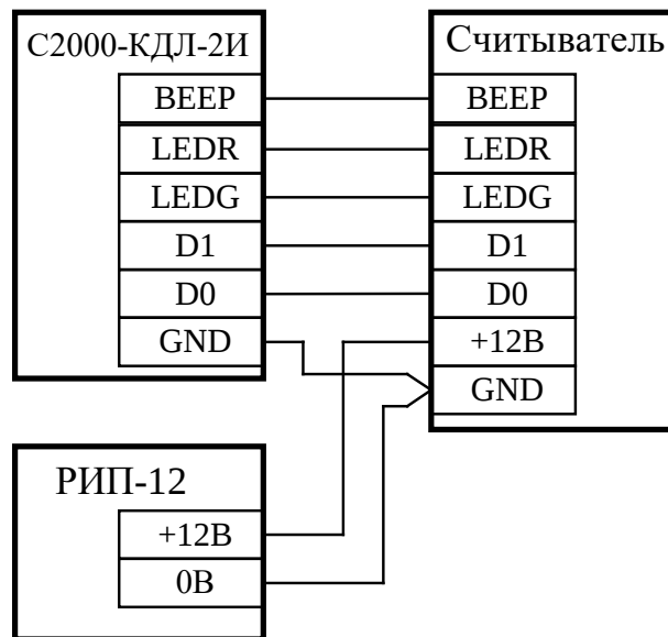
Рисунок 2.2.4.4.3 Схема подключения считывателей с интерфейсом Wiegand
