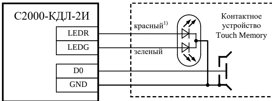
Рисунок 2.2.4.4.1 Схема подключения контактного устройства Touch Memory
