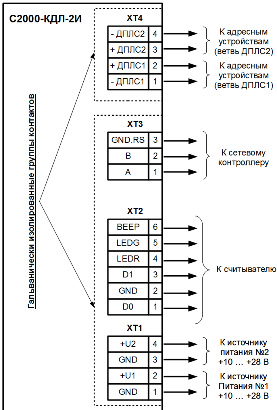
Рисунок 2.2.4.1. Схема электрическая подключения контроллера
