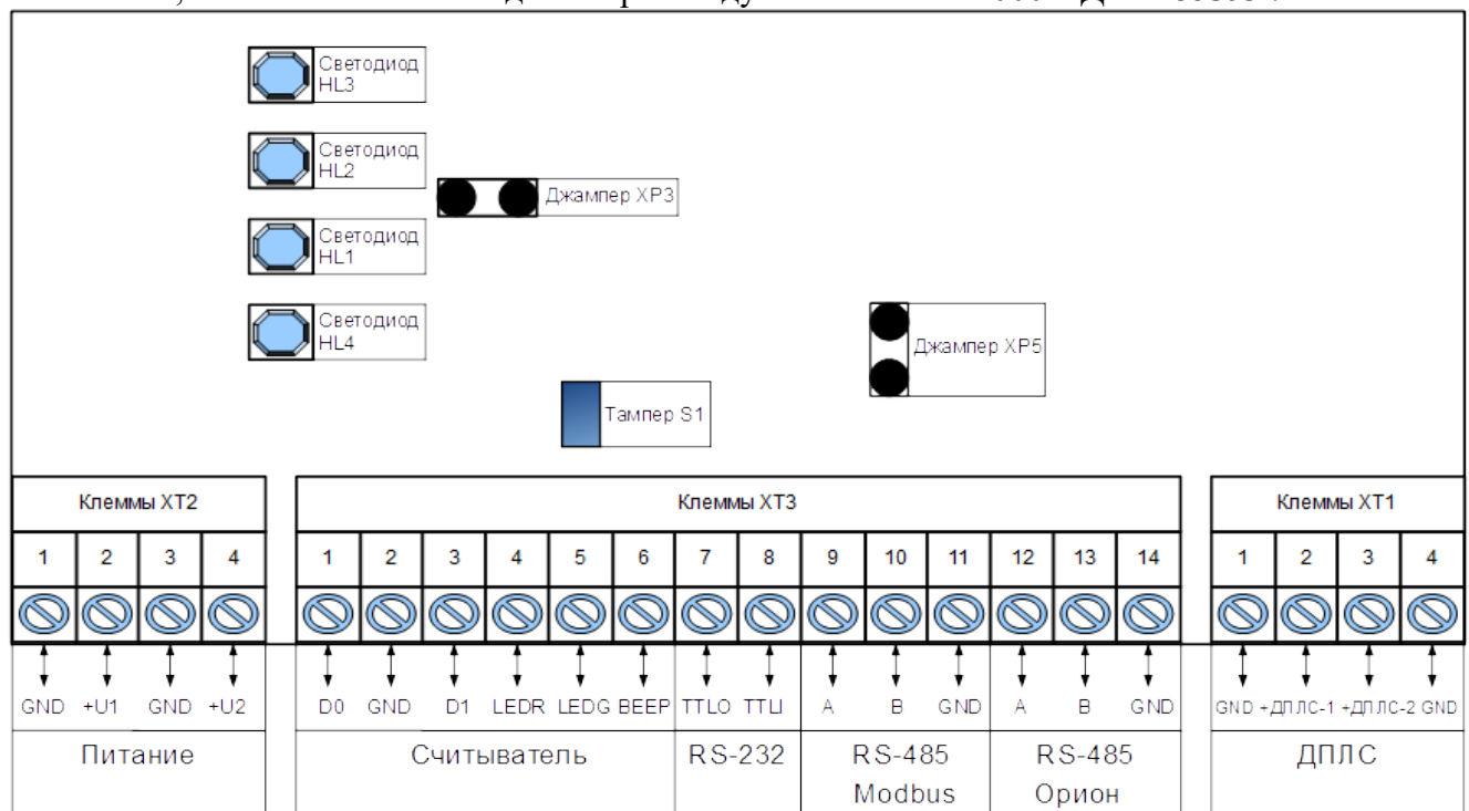
Рисунок 1. Плата модуля
