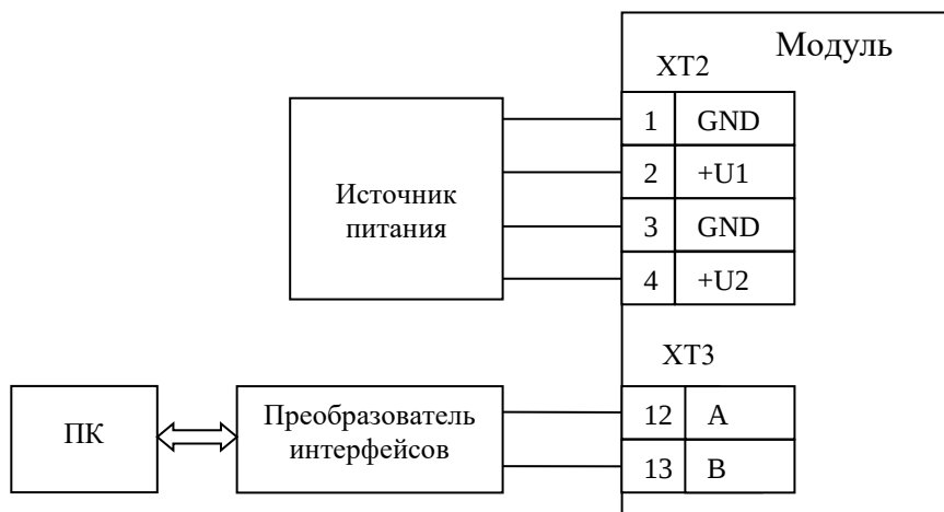
Рисунок 5. Схема для конфигурирования модуля
