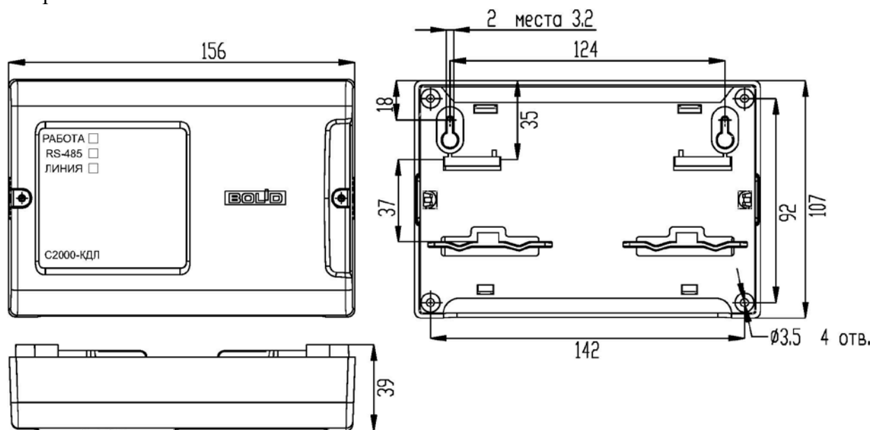
Рисунок 2.2.2.1. Габаритные и установочные размеры контроллера
