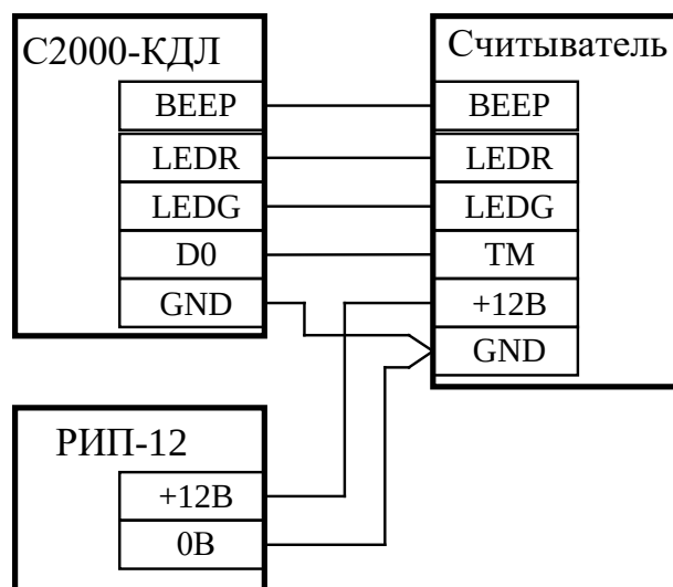
Рисунок 2.2.4.4.2. Схема подключения считывателей с интерфейсом Touch Memory
