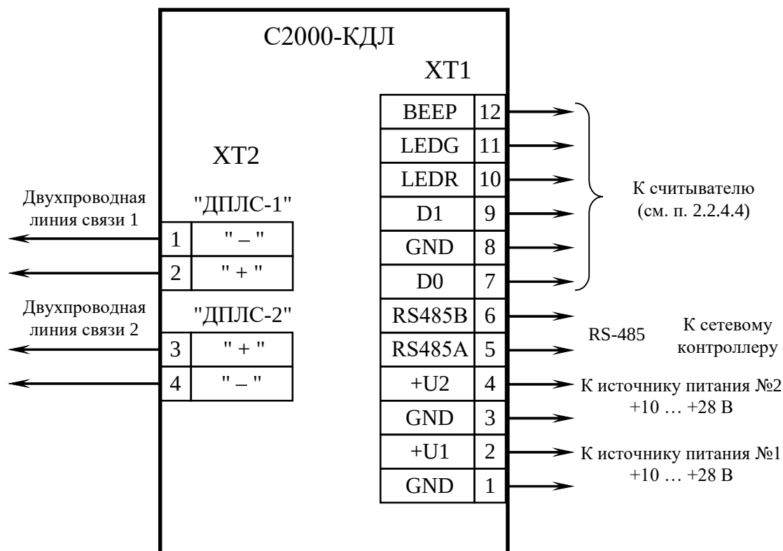
Рисунок 2.2.4.1. Схема электрическая подключения контроллера
