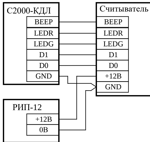
Рисунок 2.2.5 Схема подключения счетчиков с интерфейсом Wiegand
