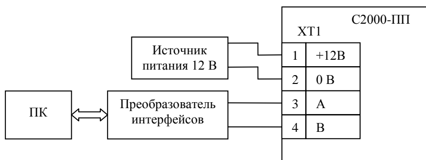
Рисунок 8. Схема для конфигурирования «С2000-ПП»
