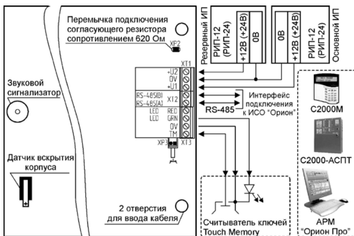
Рисунок 3. Схема внешних соединений блока «С2000-ПТ»
