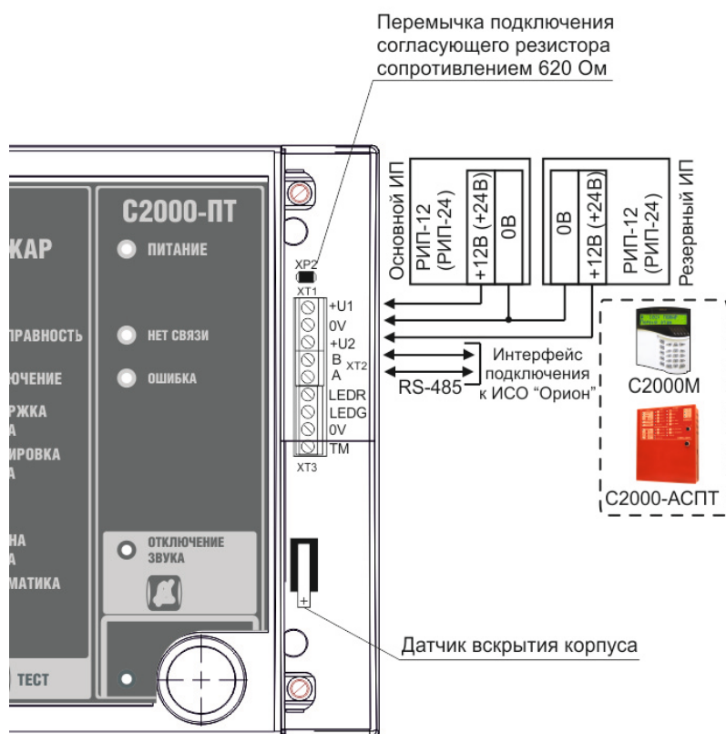
Рисунок 2. Схема внешних соединений блока «С2000-ПТ»
