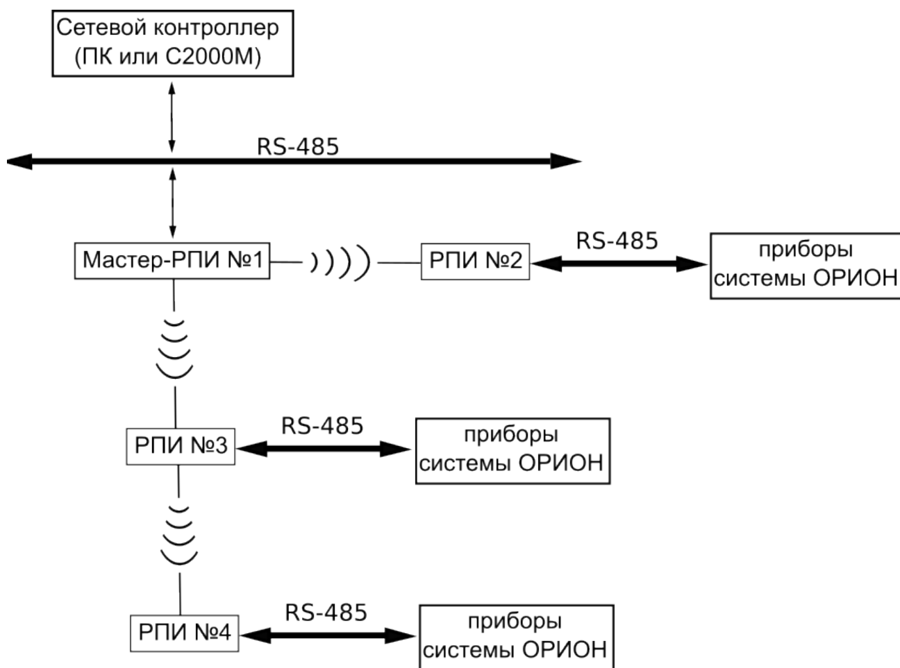
Рисунок 1.4.7.3. Пример использования ретрансляции пакетов по радиоканалу (РПИ №3 осуществляет ретрансляцию данных от РПИ №4)
