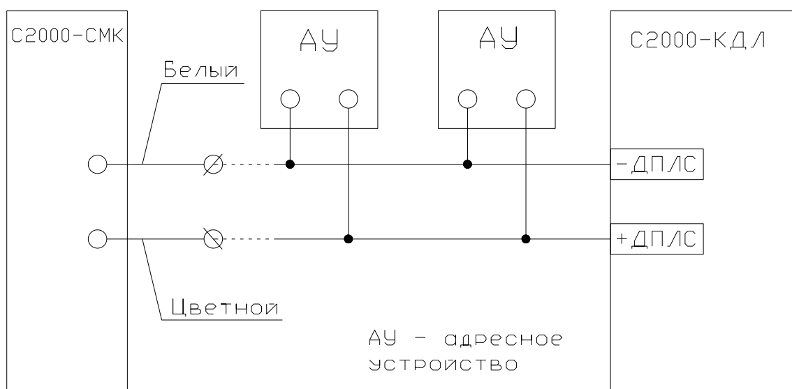
Рисунок 2.2.4.1 Схема подключения
