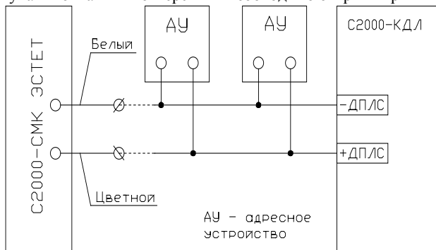
Рисунок 1 Схема соединений
