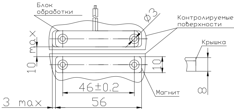
Рисунок 2 Установочные размеры
