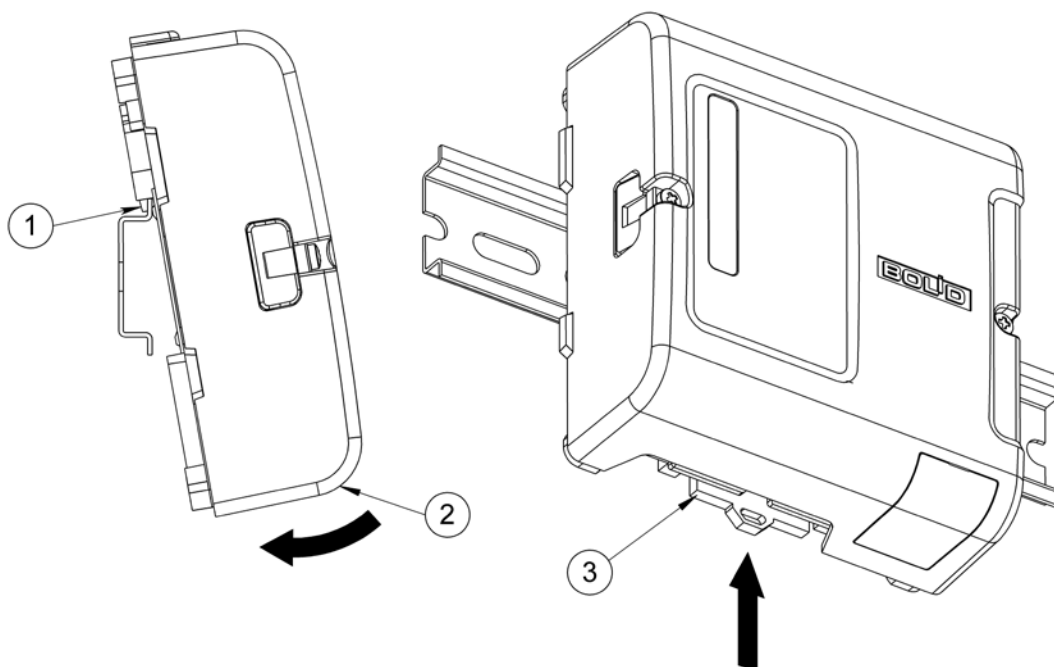
Рисунок 2.2.2 – Снятие крышки корпуса блока.
