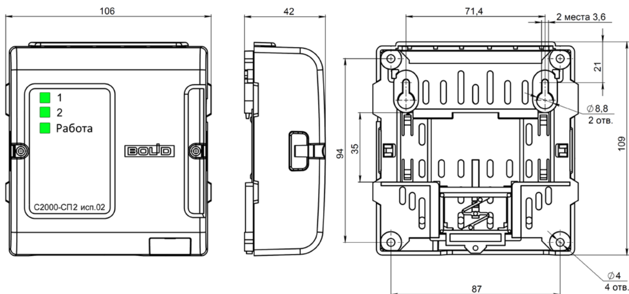
Рисунок 2.2.1 – Внешний вид и габаритно-установочные размеры блока.
