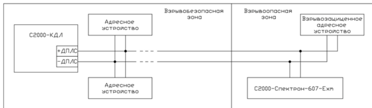
Рисунок 2.2.4.2 – Пример подключения извещателя «С2000-Спектрон-607-Ехm» к двухпроводной линии связи
