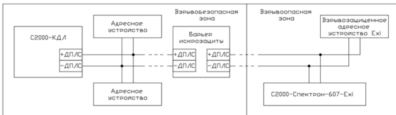
Рисунок 2.2.4.1 – Пример подключения извещателя «С2000-Спектрон-607-Ехi» к двухпроводной линии связи.
