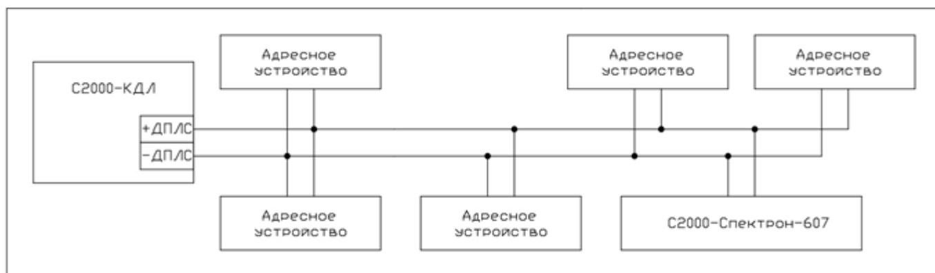
Рисунок 2.2.4.1 – Пример подключения извещателя к двухпроводной линии связи.
