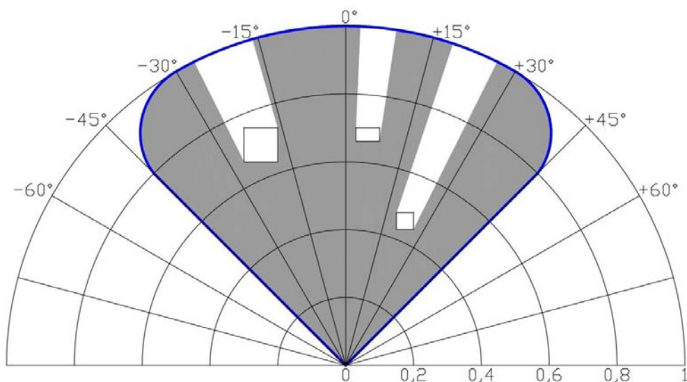
Рисунок 2.1.2.3 – Влияние посторонних предметов на зону чувствительности извещателя.
