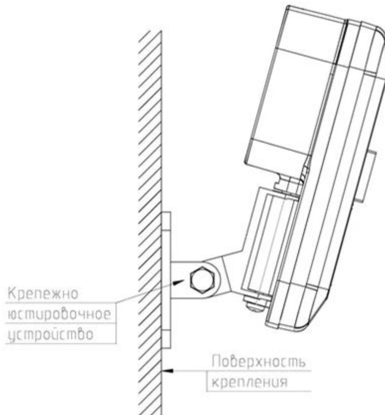
Рисунок 2.2.3.1 – Пример установки извещателя.
