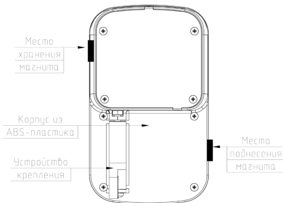
Рисунок 2.2.2.3 – Расположение основных компонентов извещателя, относительно тыловой части корпуса.
