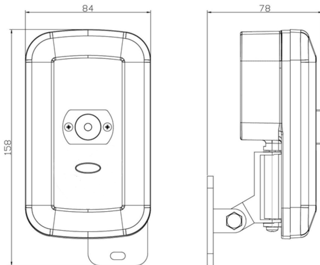
Рисунок 2.2.2.4 – Габаритные размеры извещателя «С2000-Спектрон-607».
