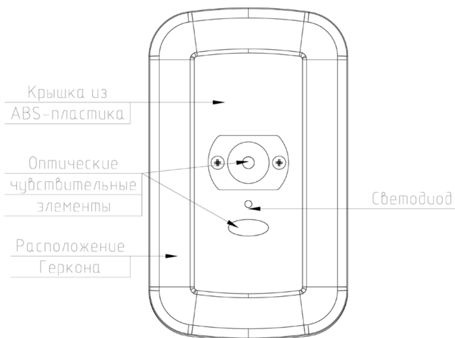
Рисунок 2.2.2.2 – Расположение основных компонентов извещателя, относительно лицевой части корпуса.
