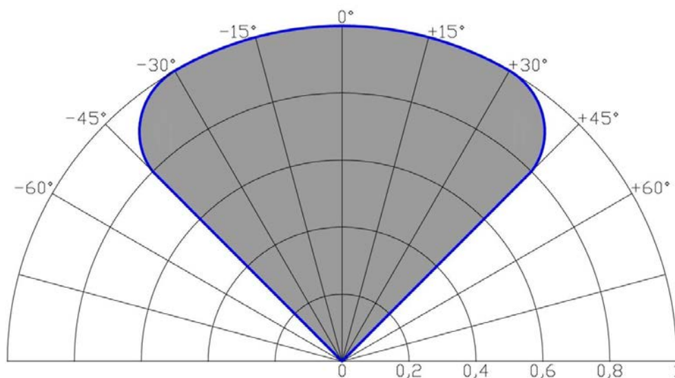
Рисунок 2.1.2.2 – Диаграмма зоны чувствительности извещателя к тестовому очагу пламени ТП-5, ТП-6.
