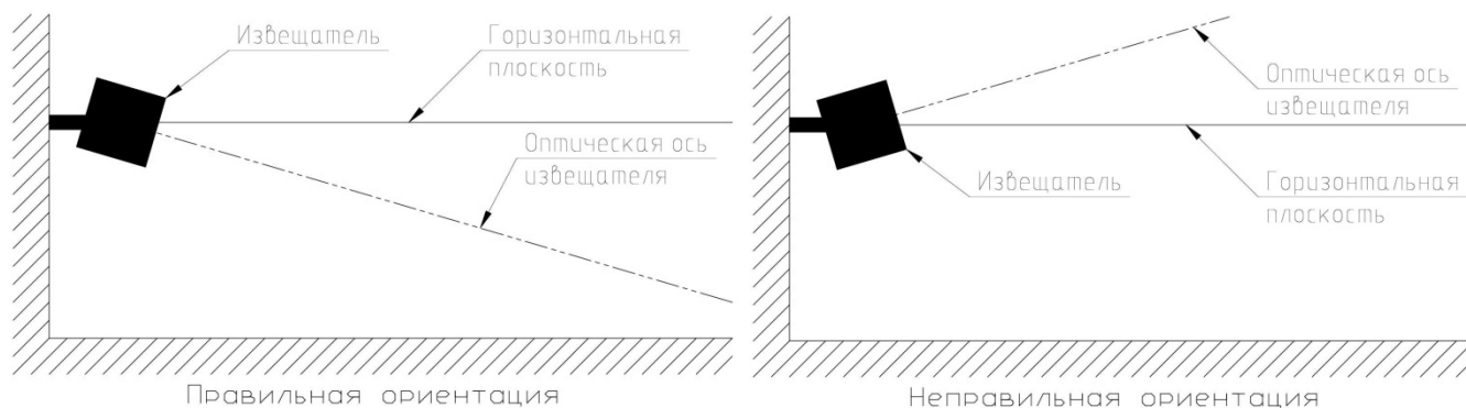
Рисунок 2.1.2.1 – Правильная и неправильная ориентация извещателя.
