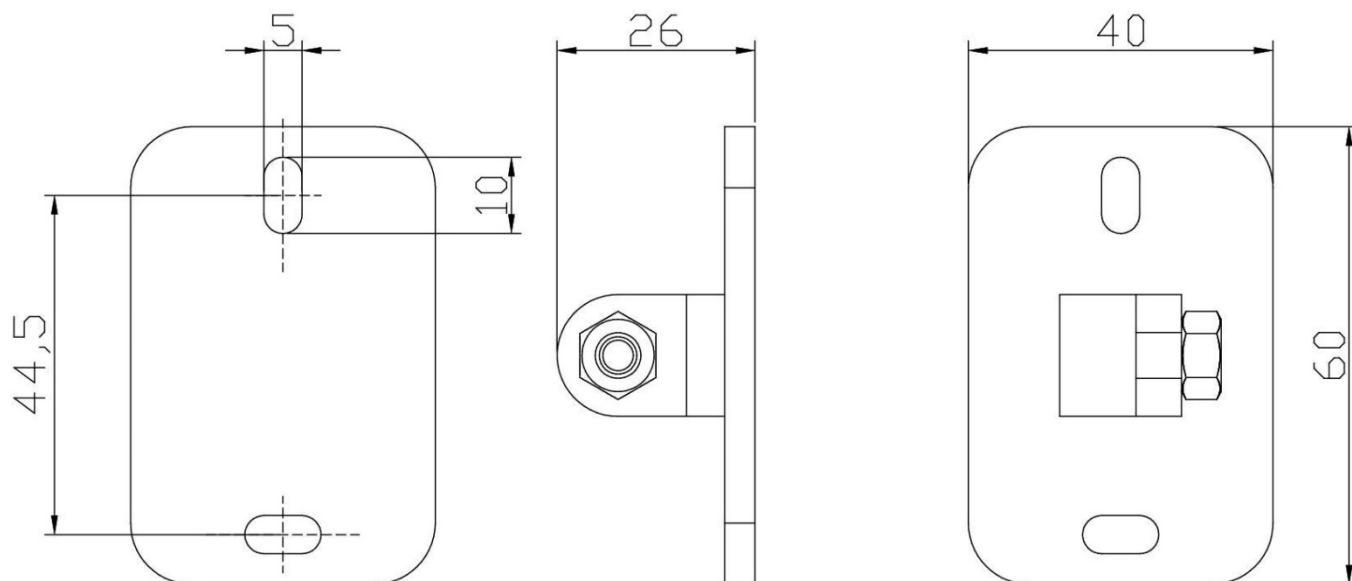
Рисунок 2.2.2.5 – Габаритные и установочные размеры крепления извещателя «С2000-Спектрон-607».
