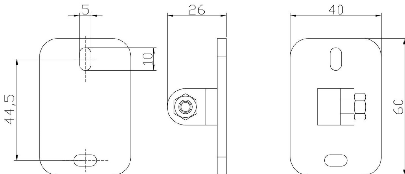
Рисунок 2.2.2.5 – Габаритные и установочные размеры крепления извещателя.
