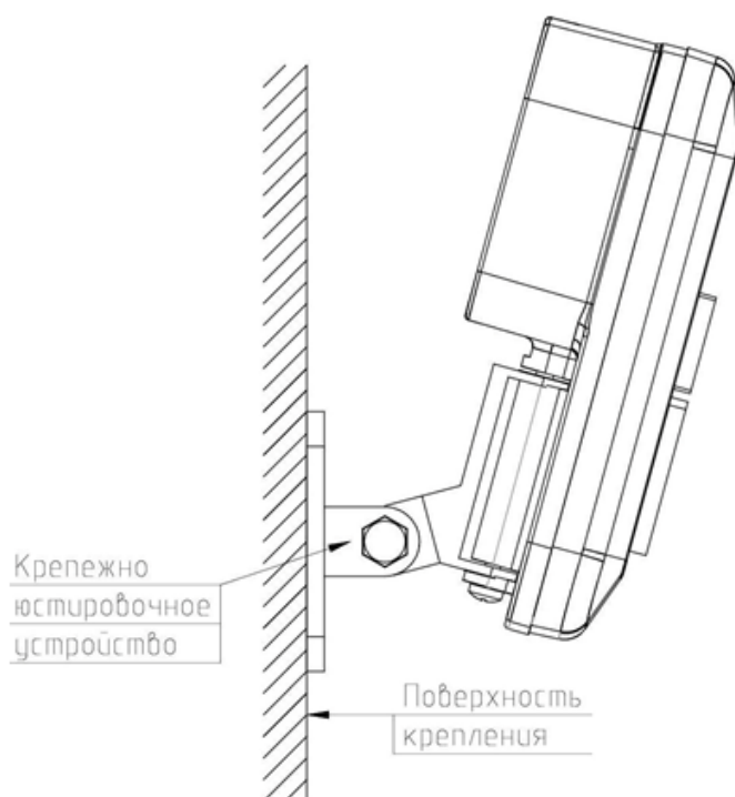
Рисунок 2.2.3.1 – Пример установки извещателя.
