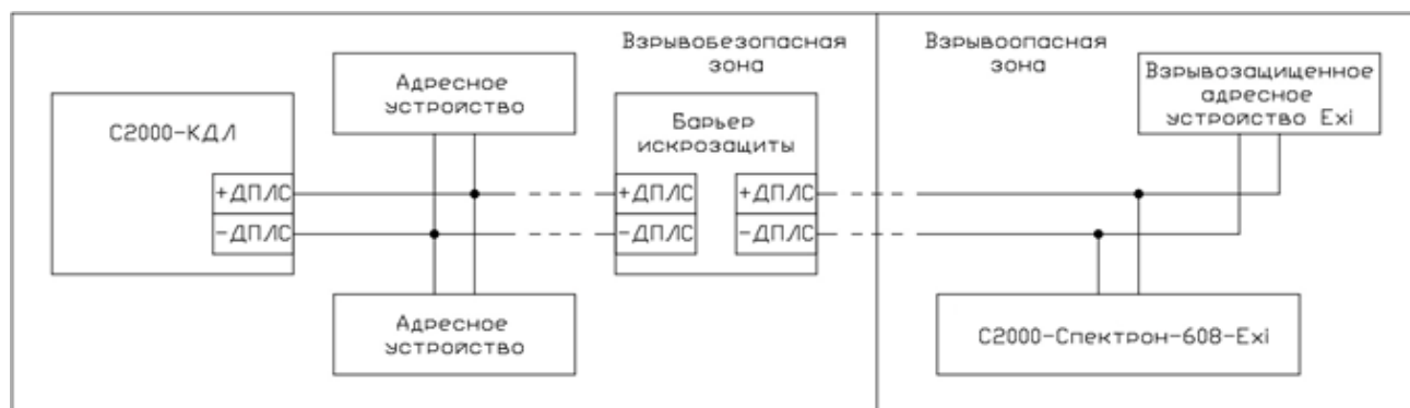
Рисунок 2.2.4.1 – Пример подключения извещателя «С2000-Спектрон-608-Ехi» к двухпроводной линии связи.
