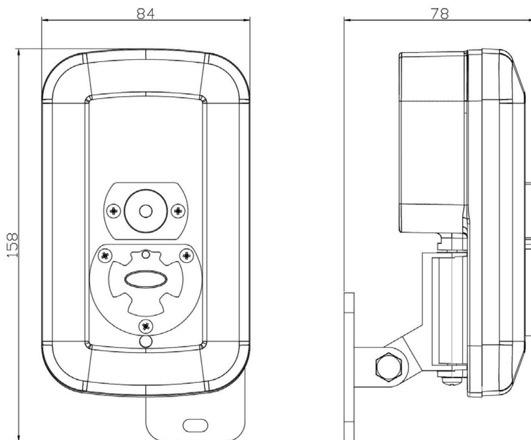
Рисунок 2.2.2.4 – Габаритные размеры извещателя
