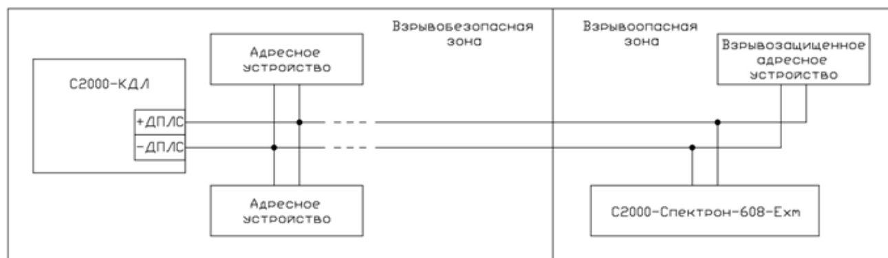
Рисунок 2.2.4.2 – Пример подключения извещателя «С2000-Спектрон-608-Ехm» к двухпроводной линии связи
