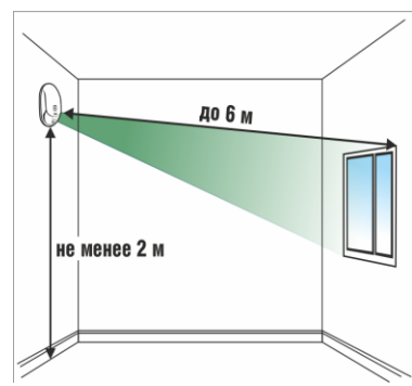
Рисунок 2.2.3.2.3 Установка извещателя на противоположной стене
