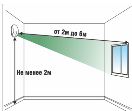
Рисунок 2.2.3.2.3 Установка извещателя на противоположной стене
