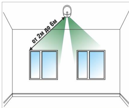
Рисунок 2.2.3.2.1 Установка извещателя на потолке
