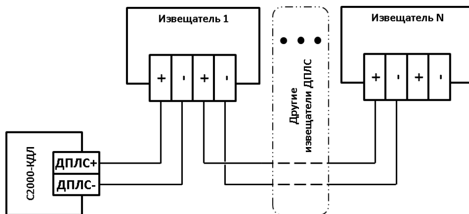
Рис.2.2.4.1 Схема подключения извещателя к контроллеру КДЛ
