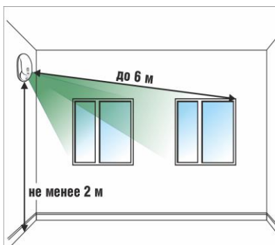
Рисунок 2.2.3.2.2 Установка извещателя на боковой стене
