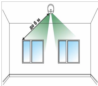
Рисунок 2.2.3.2.1 Установка извещателя на потолке
