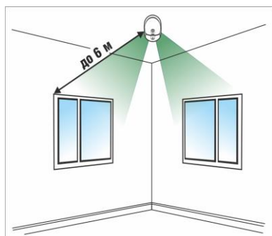
Рисунок 2.2.3.2.4 Установка извещателя для блокировки оконных проемов в соседних стенах
