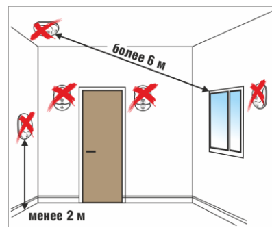
Рисунок 2.2.3.2.6 Не рекомендуемые места установки извещателя
