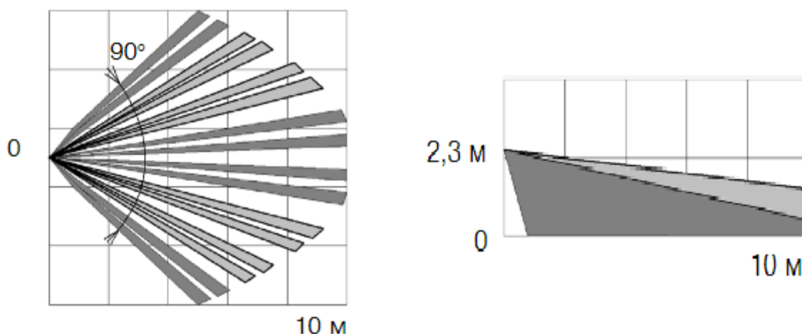
Рисунок 2.4 Зона обнаружения
