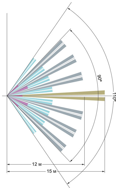
Рисунок 2.4 Зона обнаружения
