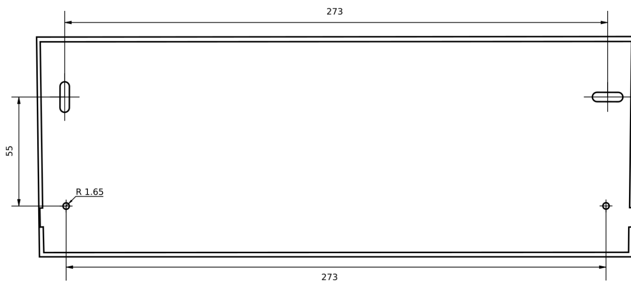
Рисунок 2.4 Монтажные размеры
