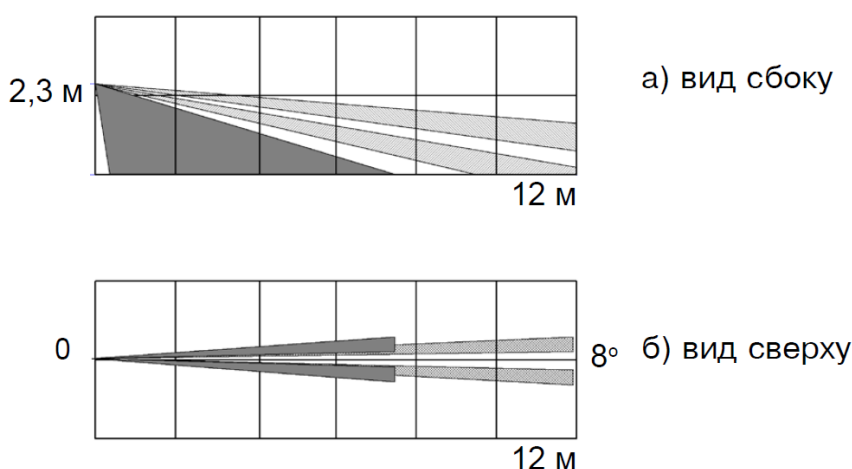
Рисунок 2.5 Зона обнаружения
