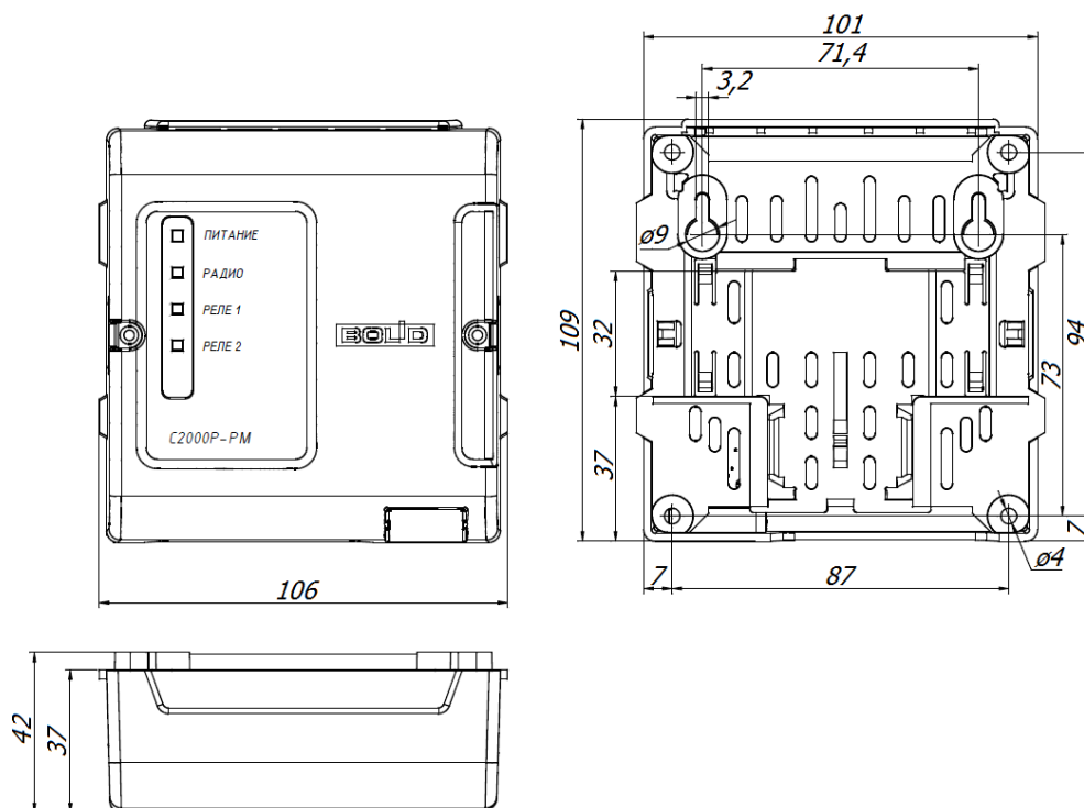
Рисунок 2.4 Монтажные размеры
