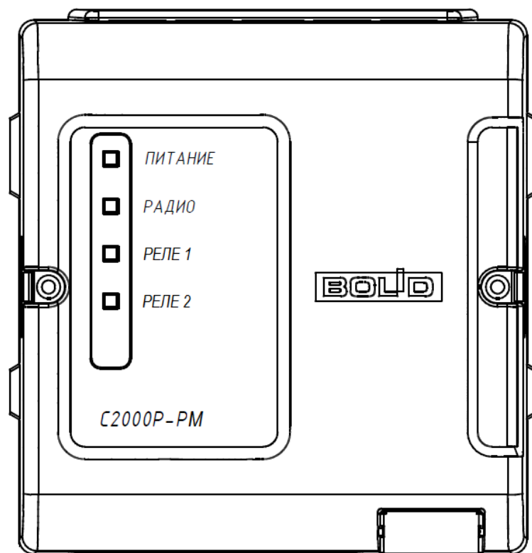
Рисунок 2.1 Внешний вид
