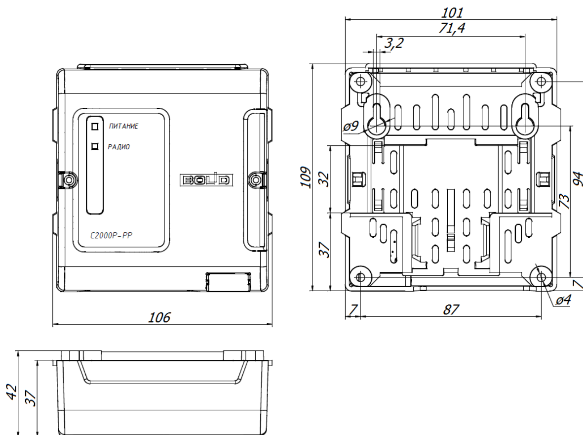
Рисунок 2.2.2.3.1 Монтажные размеры
