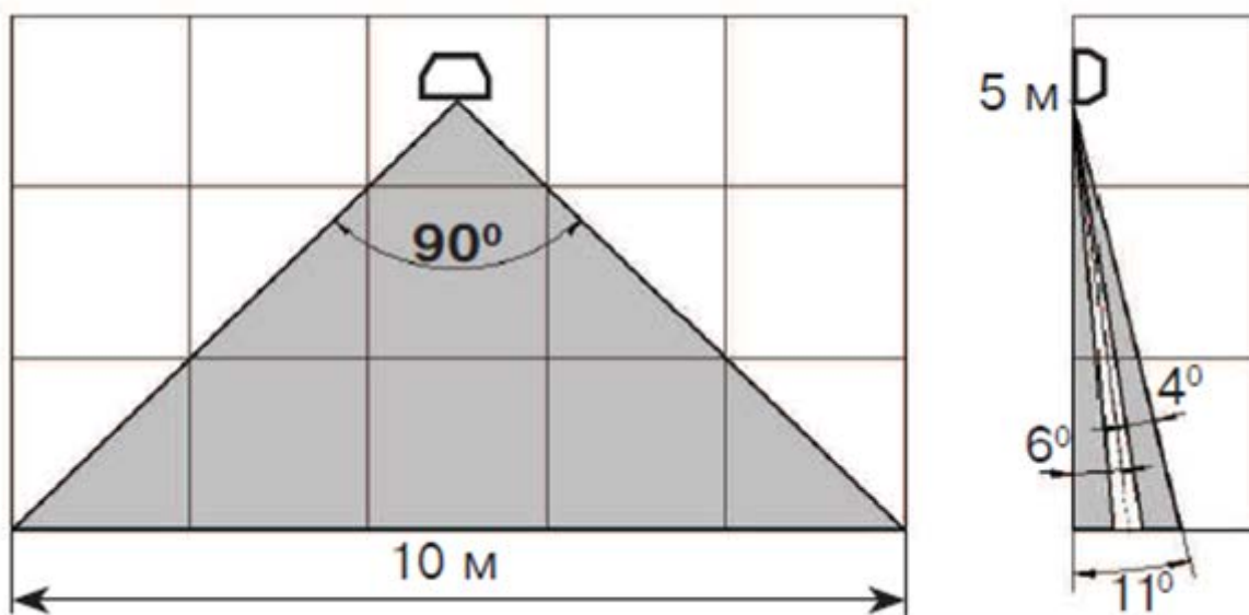
Рисунок 2.4 Зона обнаружения
