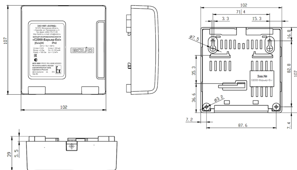
Рисунок 2.2.2.1. Габаритный чертёж барьера.
