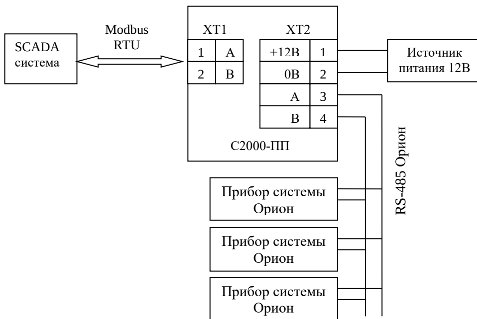
Рисунок 17. Подключение «С2000-ПП» в режиме «Орион-Master»
