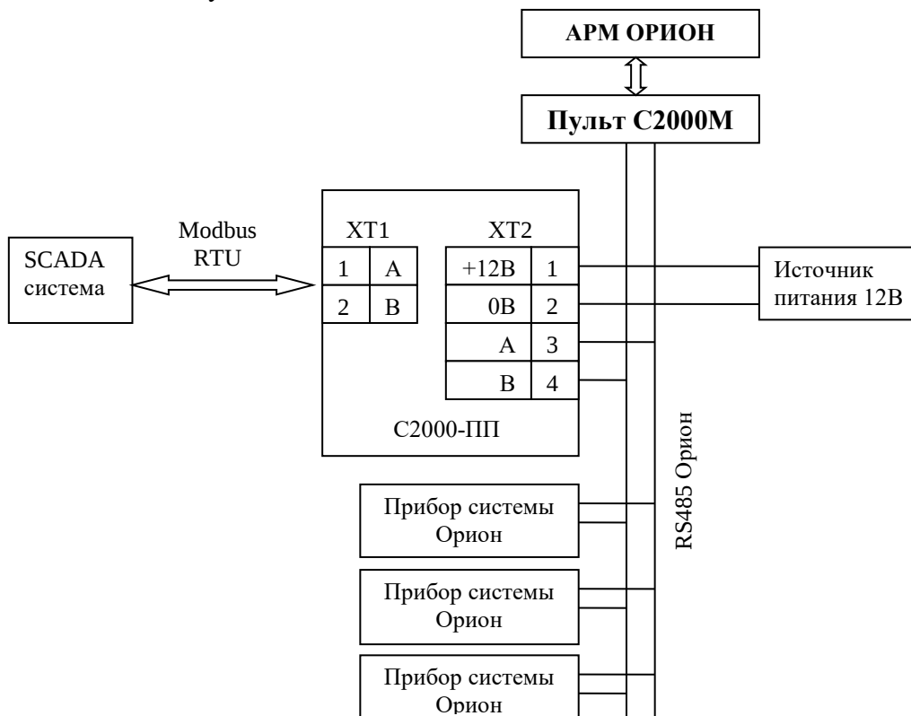
Рисунок 18. Подключение «С2000-ПП» в режиме «Орион-Slave»
