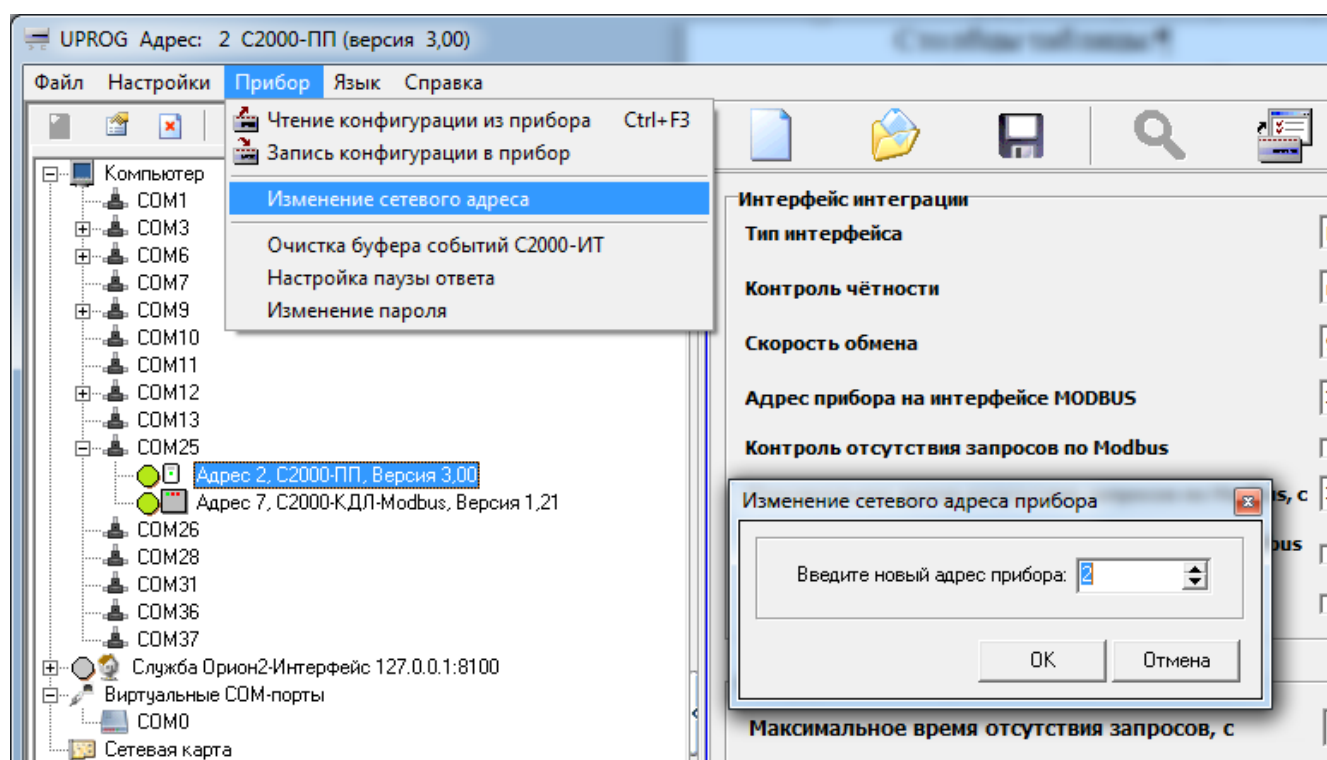
Рисунок 13. Изменение адреса прибора на интерфейсе Орион.
