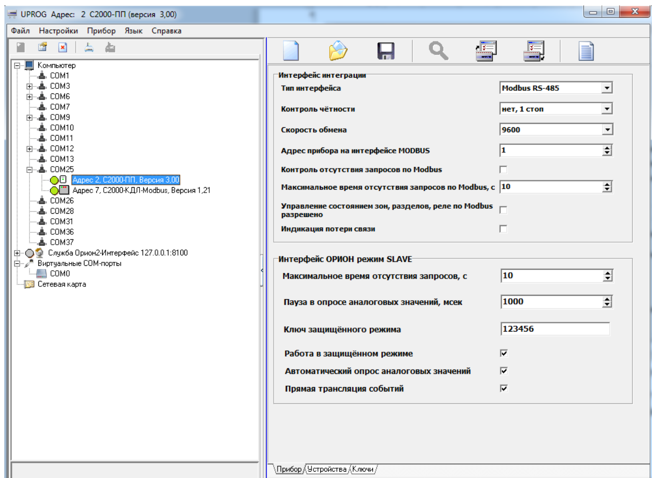
Рисунок 7. Конфигурационные параметры. Страница «Прибор»
