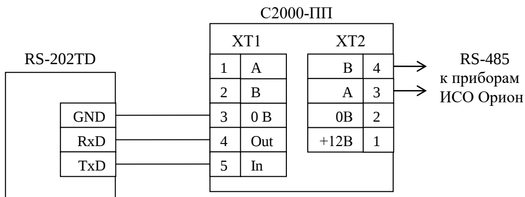
Рисунок 19. Подключение передатчика к «С2000-ПП»
