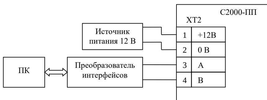
Рисунок 5. Схема для конфигурирования «С2000-ПП»
