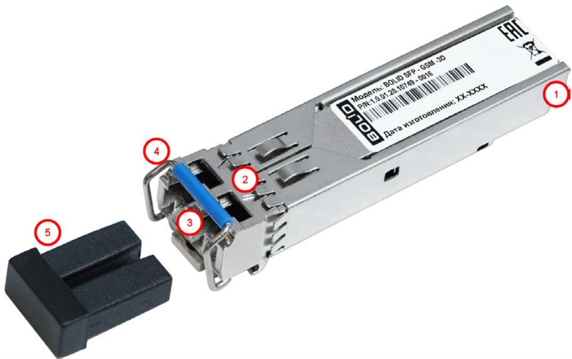
Рисунок 4.1 – Устройство SFP-модуля
