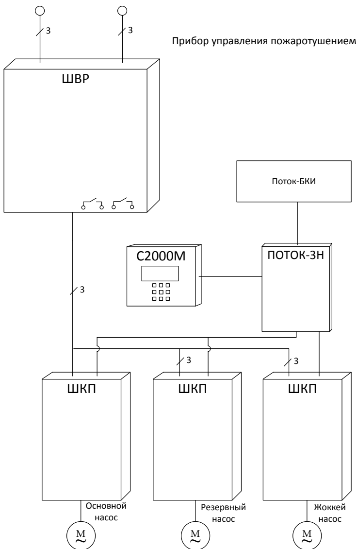
Рисунок 1. Схема питания ШКП в составе ППУ.
