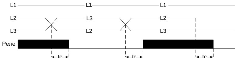
Рисунок 5. Контроль порядка чередования и обрыва фаз
