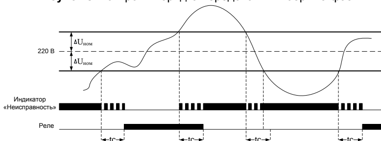
Рисунок 6. Контроль напряжения фазы
