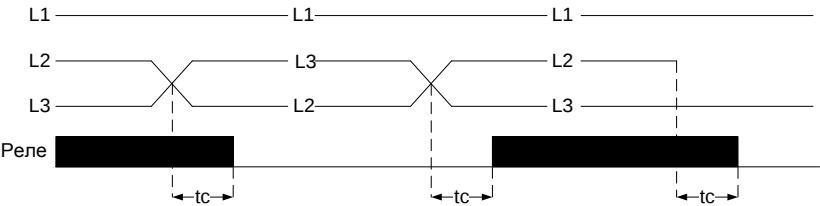
Рисунок 5. Контроль порядка чередования и обрыва фаз
