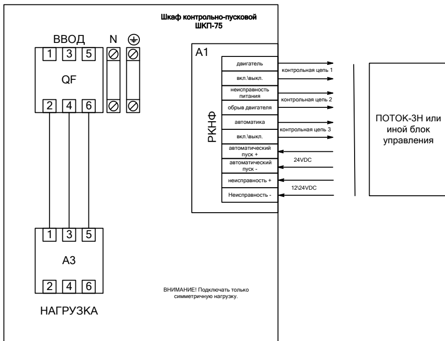
Рисунок 3. Схема электрическая подключения шкафа при эксплуатации
