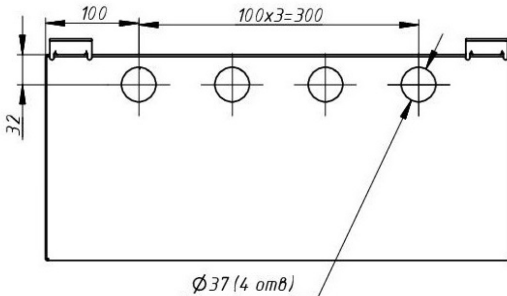
Вид корпуса сверху
