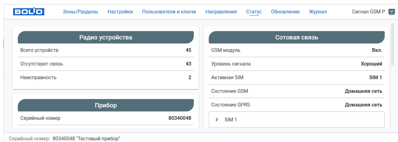
Рисунок 2.4-1 Общий вид WEB-интерфейса
