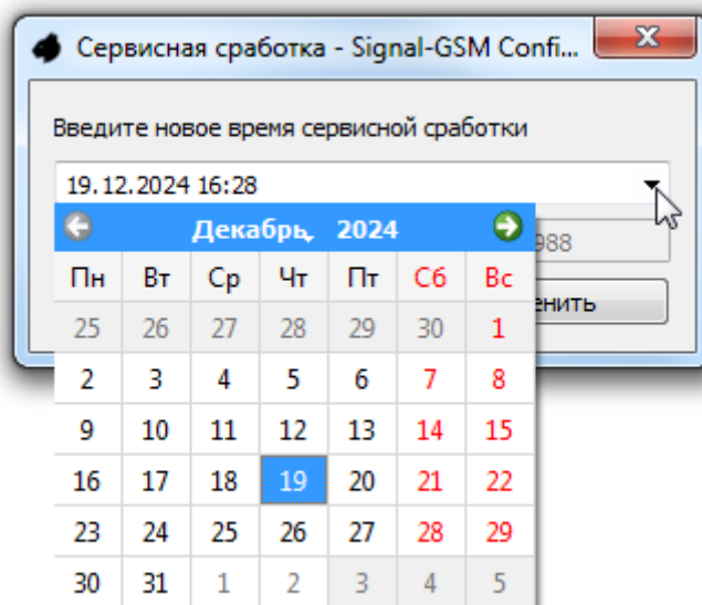
Рисунок 2.3.8.11.3-3 Задание даты и времени сервисной сработки
