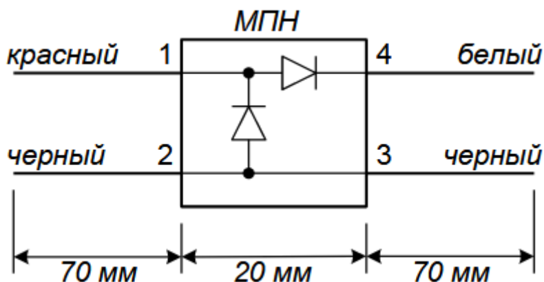
Рисунок 2.2.4.4-1 Схема модуля подключения нагрузки (МПН)
