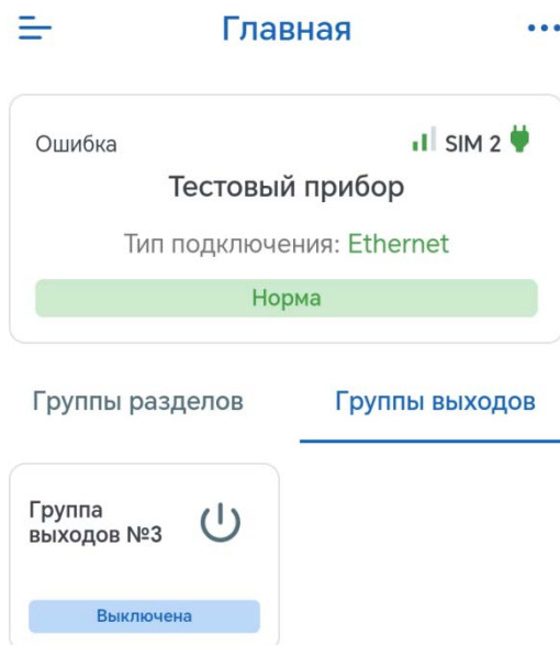
Рисунок 2.4.4.5-1 Управление выходами
