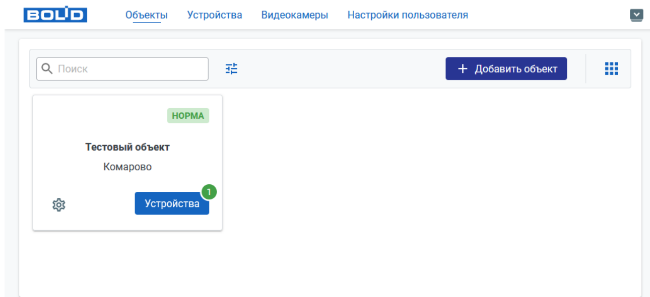
Рисунок 2.4.2.5.1-3 Добавленный Объект
