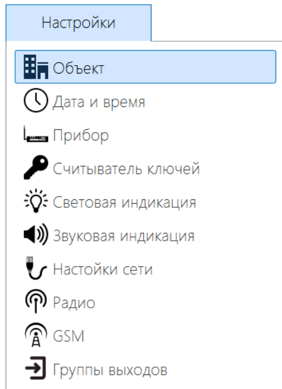
Рисунок 2.3.3-1 Группы настроек
