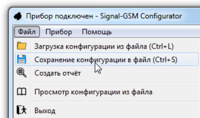
Рисунок 2.3.14.1-1 Меню «Файл»
