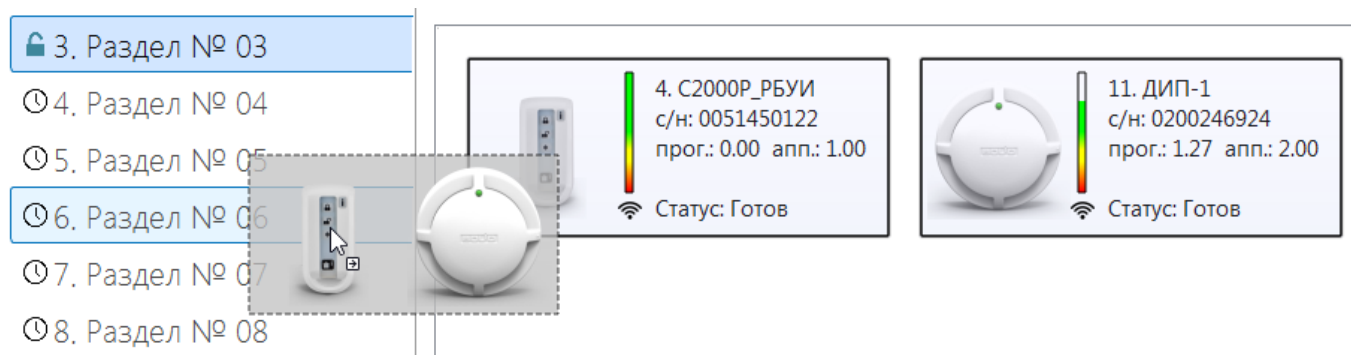
Рисунок 2.3.5.5-1 Перемещение РУ
