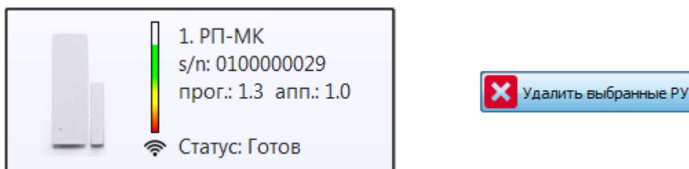
Рисунок 2.3.5.4-1 Удаление РУ
