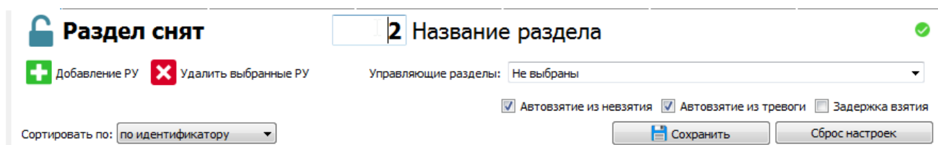
Рисунок 2.3.5.6-1 Настройки раздела
