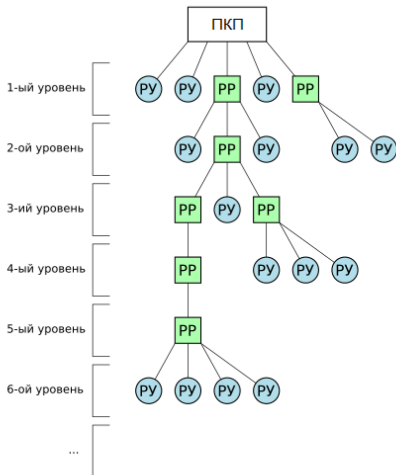
Рисунок 1.4.2-1 Цепь ретрансляции
