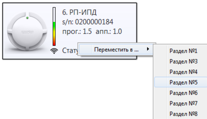
Рисунок 2.3.5.5-2 Перемещение РУ
