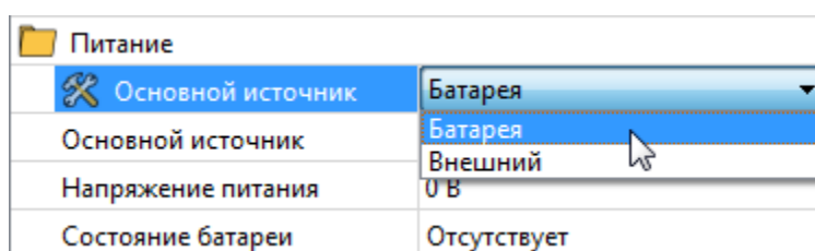
Рисунок 2.3.9.5.1-1 Настройки C2000P-PM
