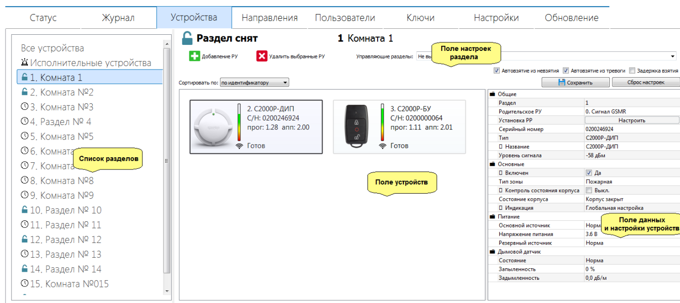
Рисунок 2.3.5-1 Вкладка «Устройства»
