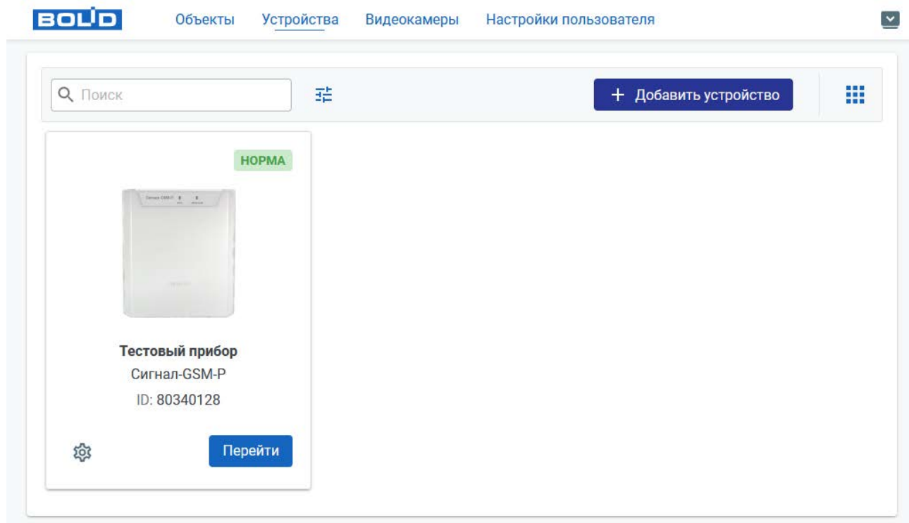
Рисунок 2.4.3.3-3 Зарегистрированный прибор
