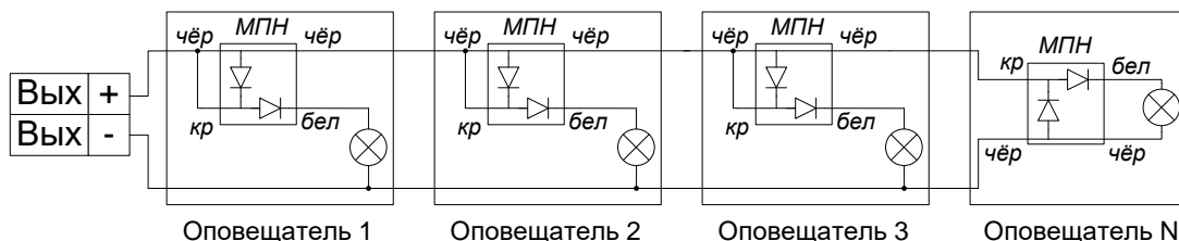
Рисунок 62. Схема подключения нескольких сирен или световых табло
