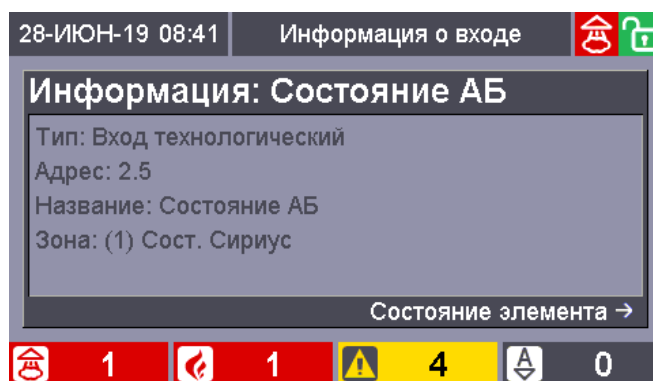
Рисунок 13. Экран режима отображения конфигурационных параметров элемента
