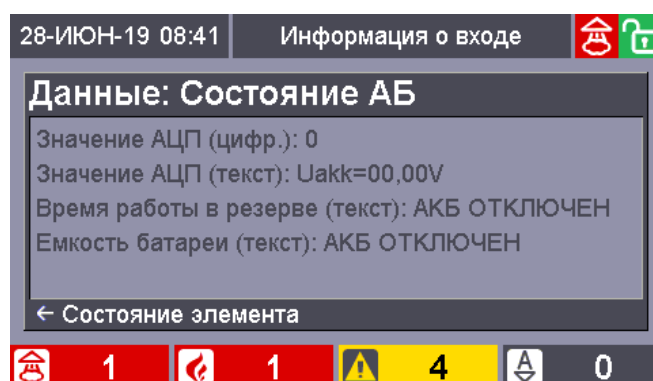
Рисунок 15. Экран режима отображения измеряемых элементом величин
