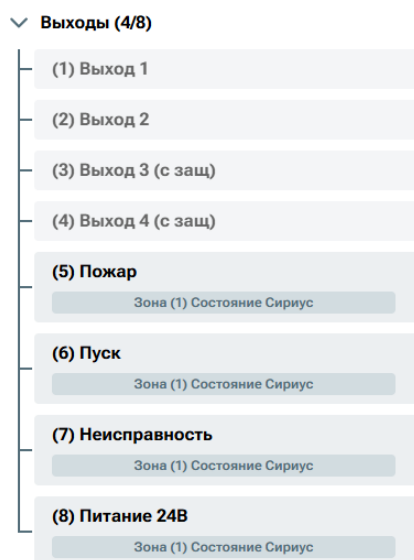
Рисунок 34. Список выходов блока «С2000-КПБ-С»
