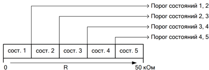
Рисунок 71. Состояния и пороги переходов между состояниями входа «Неисправность»
