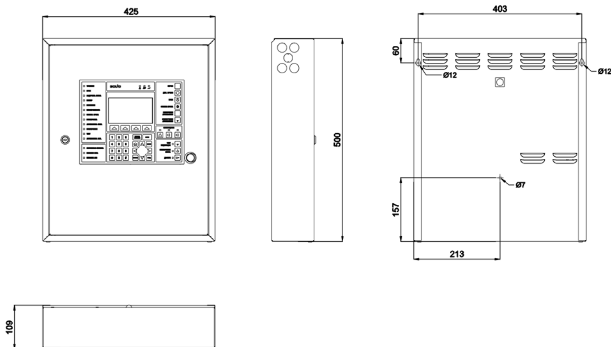
Рисунок 58. Габаритные и установочные размеры
