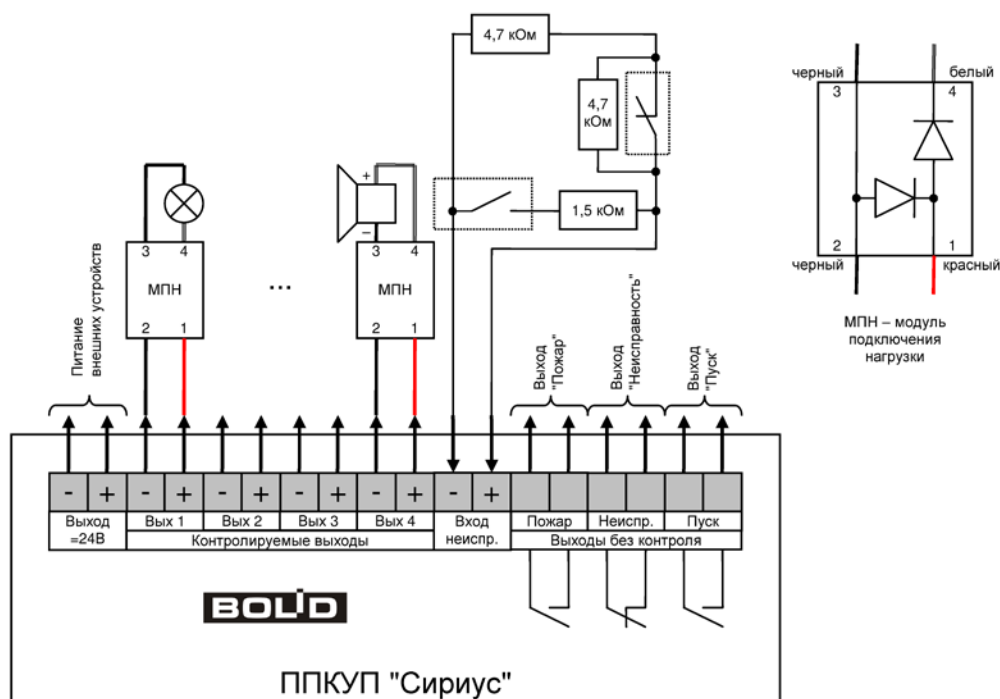
Рисунок 60. Схема подключения дискретных входов и выходов
