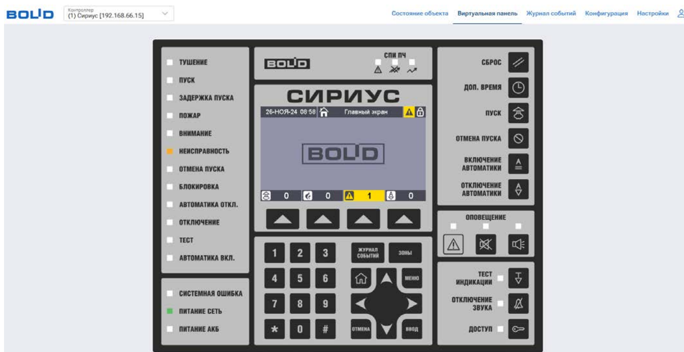
Рисунок 57. Содержимое раздела «Виртуальная панель» web-интерфейса
