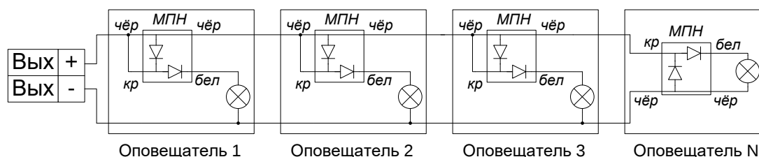
Рисунок 62. Схема подключения нескольких сирен или световых табло
