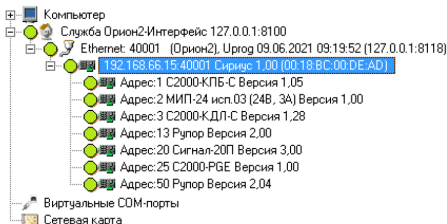
Рисунок 70. Дерево приборов в программе UProg
