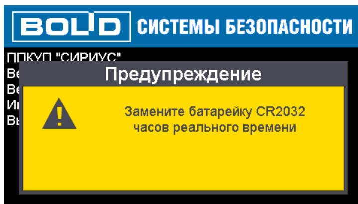
Рисунок 75. Режим предупреждения о неисправности
