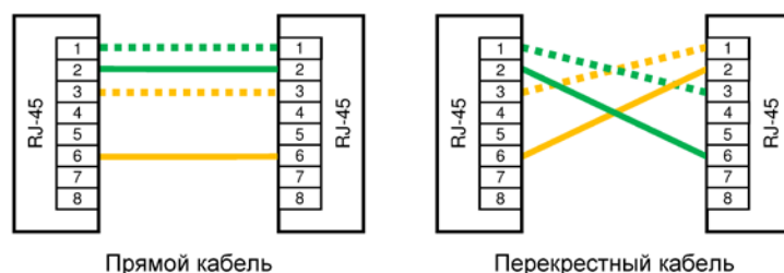
Рисунок 63. Типы Ethernet-кабелей стандарта 100BASE-TX
