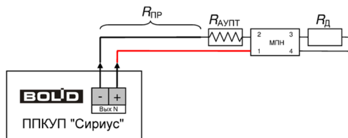
Рисунок 61. Рекомендуемая схема подключения АУП
