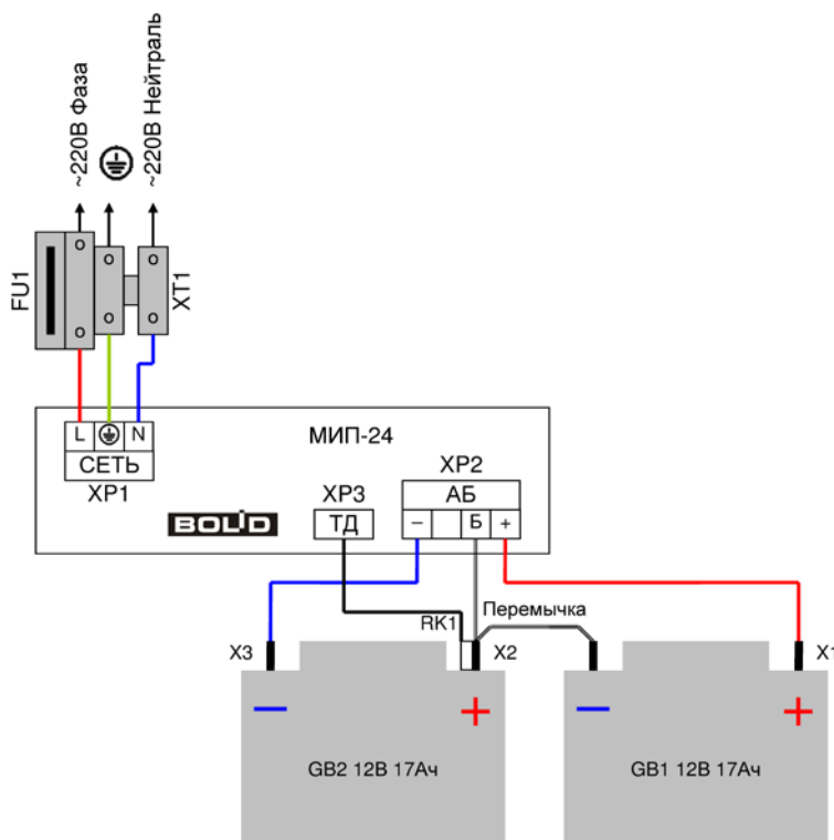
Рисунок 69. Схема подключения источников питания
