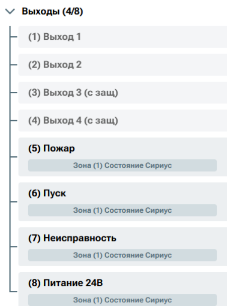
Рисунок 34. Список выходов блока «С2000-КПБ-С»
