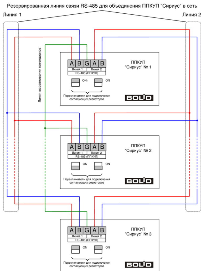
Рисунок 68. Схема объединения приборов «Сириус» в сеть
