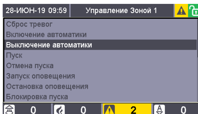
Рисунок 76. Меню выбора команды управления зоной
