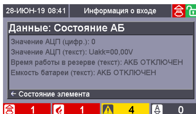
Рисунок 15. Экран режима отображения измеряемых элементом величин
