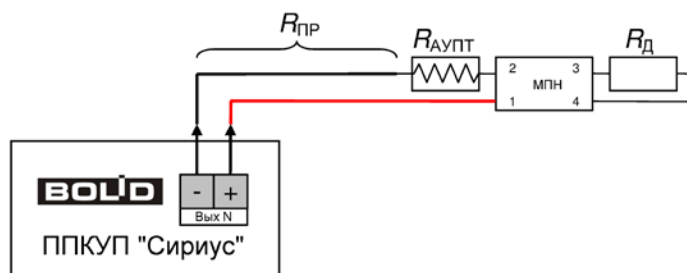
Рисунок 64. Рекомендуемая схема подключения АУП
