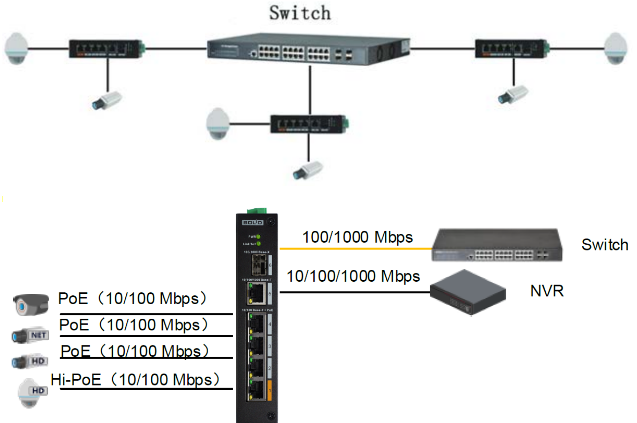
Рисунок 1.1 – Сетевое соединение
