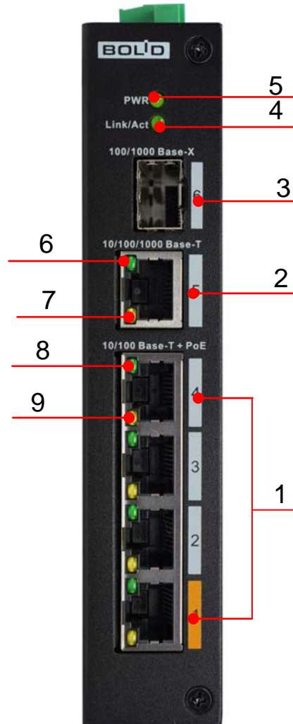
Рисунок 4.2 – Передняя панель
