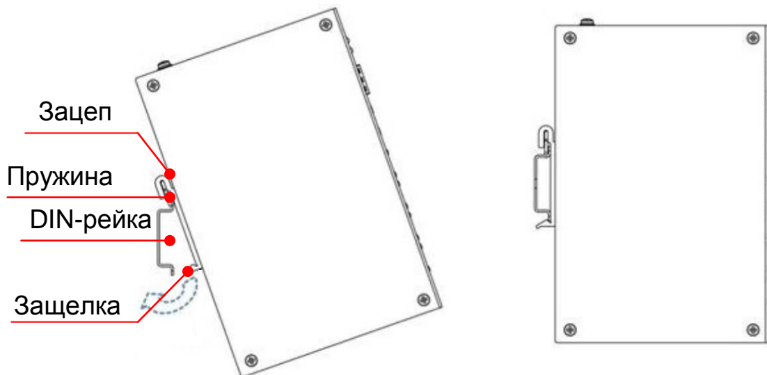
Рисунок 5.2 – Инсталляция
