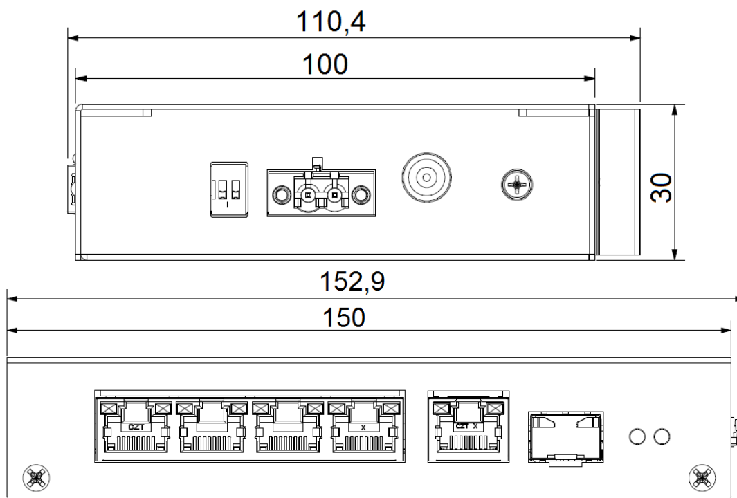
Рисунок 5.1 – Габаритные размеры
