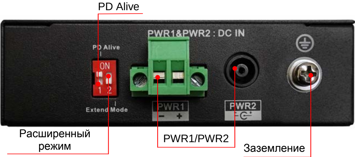
Рисунок 4.1 – Верхняя панель
