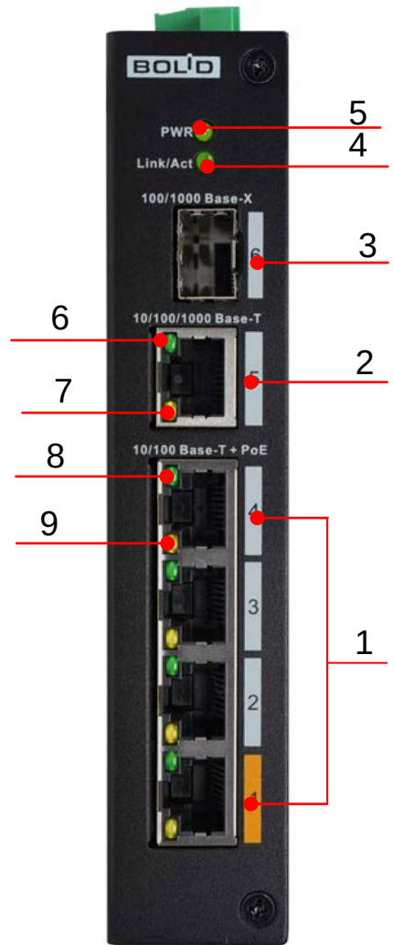
Рисунок 4.2 – Передняя панель
