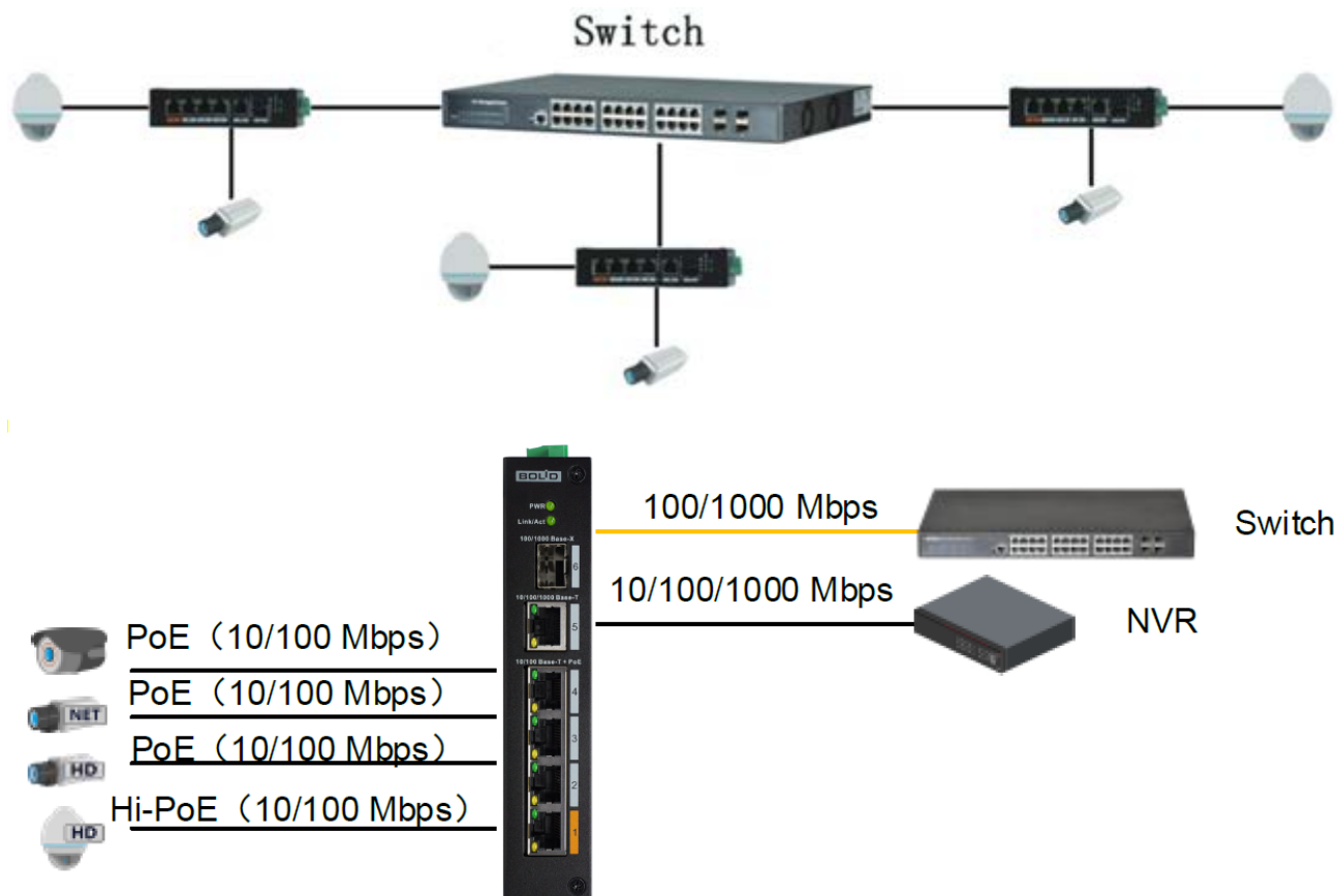
Рисунок 1.1 – Сетевое соединение
