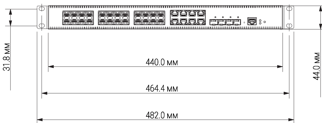
Рисунок 5.2 – Габаритные размеры
