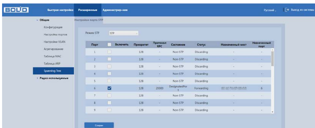
Рисунок 9.9 – Настройка STP
